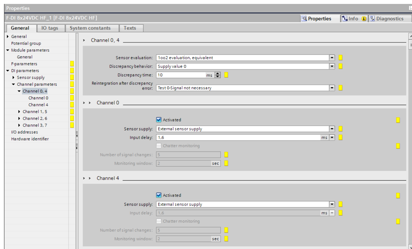
Bild 2: Parametrierung der Eingänge
