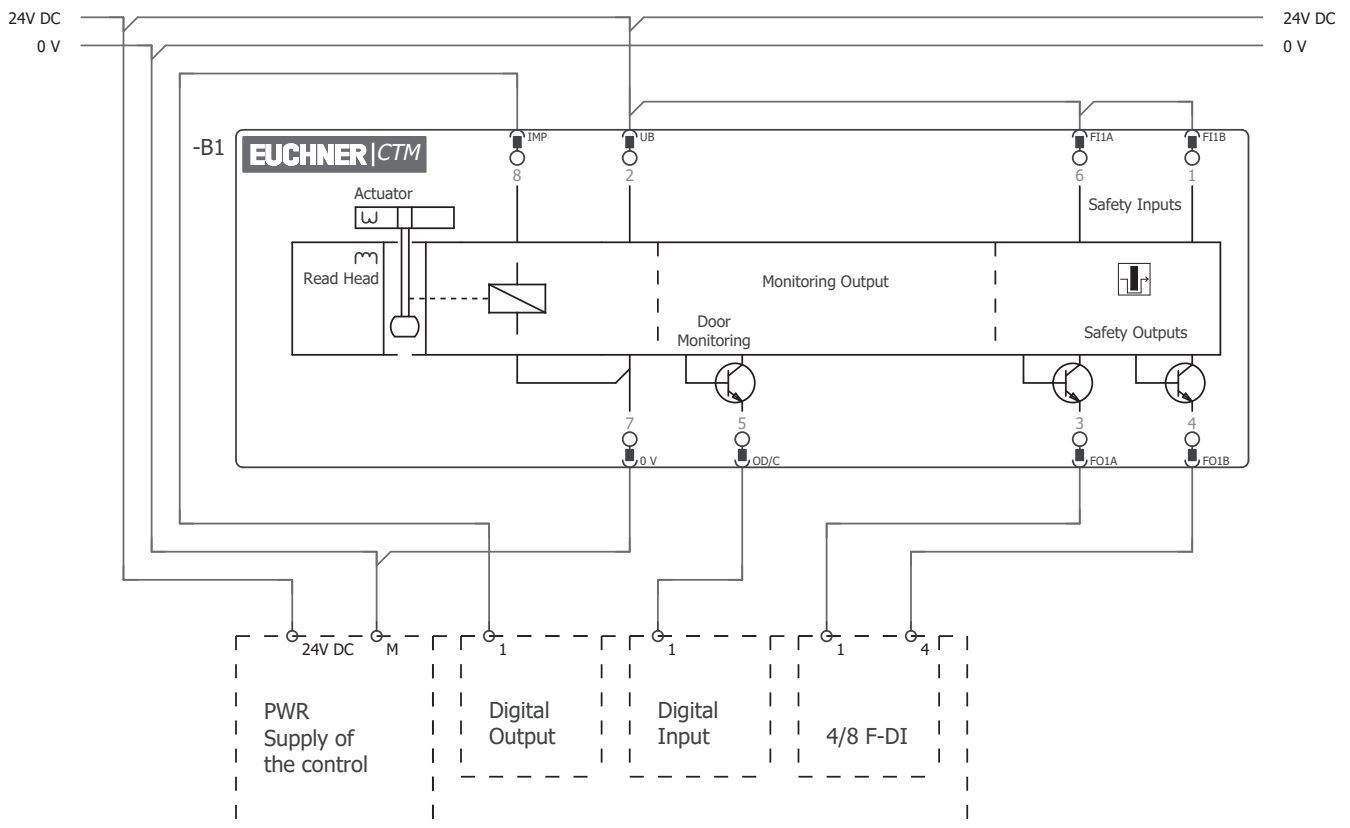
Bild 1: Prinzipielles Schaltbild CTM-LBI-BR..
