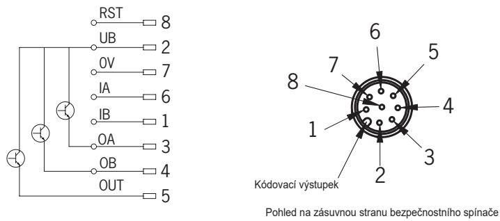
Obr. 2: Obsazení konektoru bezpečnostního spínače CES-AR
