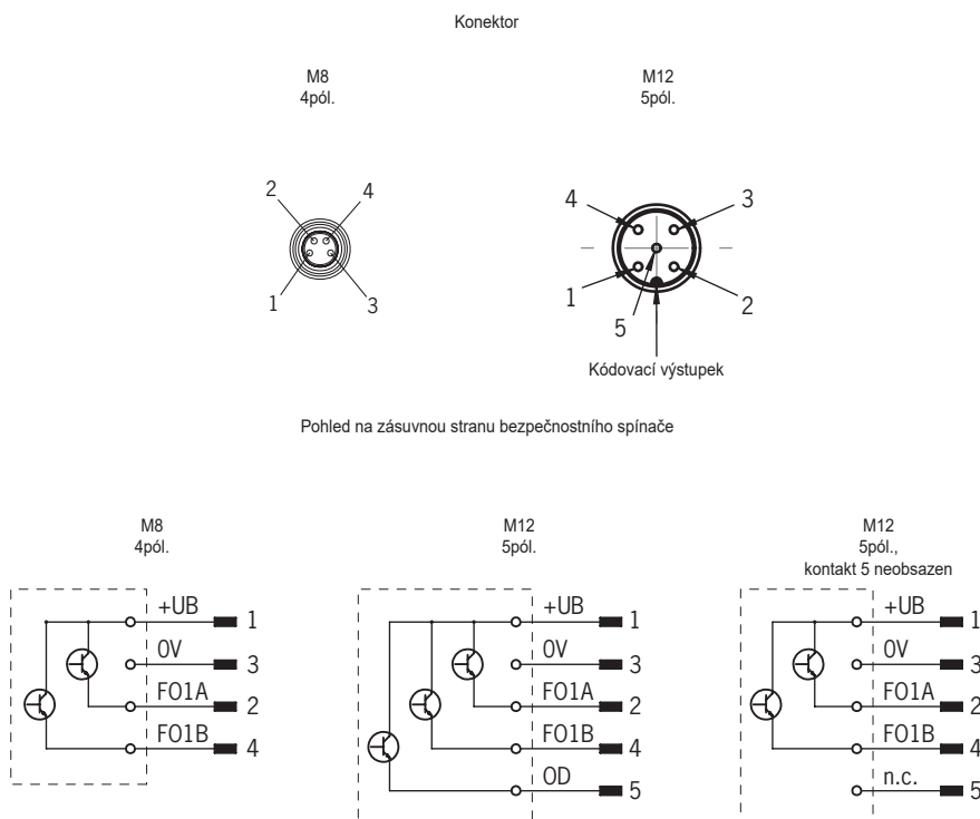
Obr. 1: Obsazení konektoru bezpečnostního spínače CES-I-AP-.-C04
