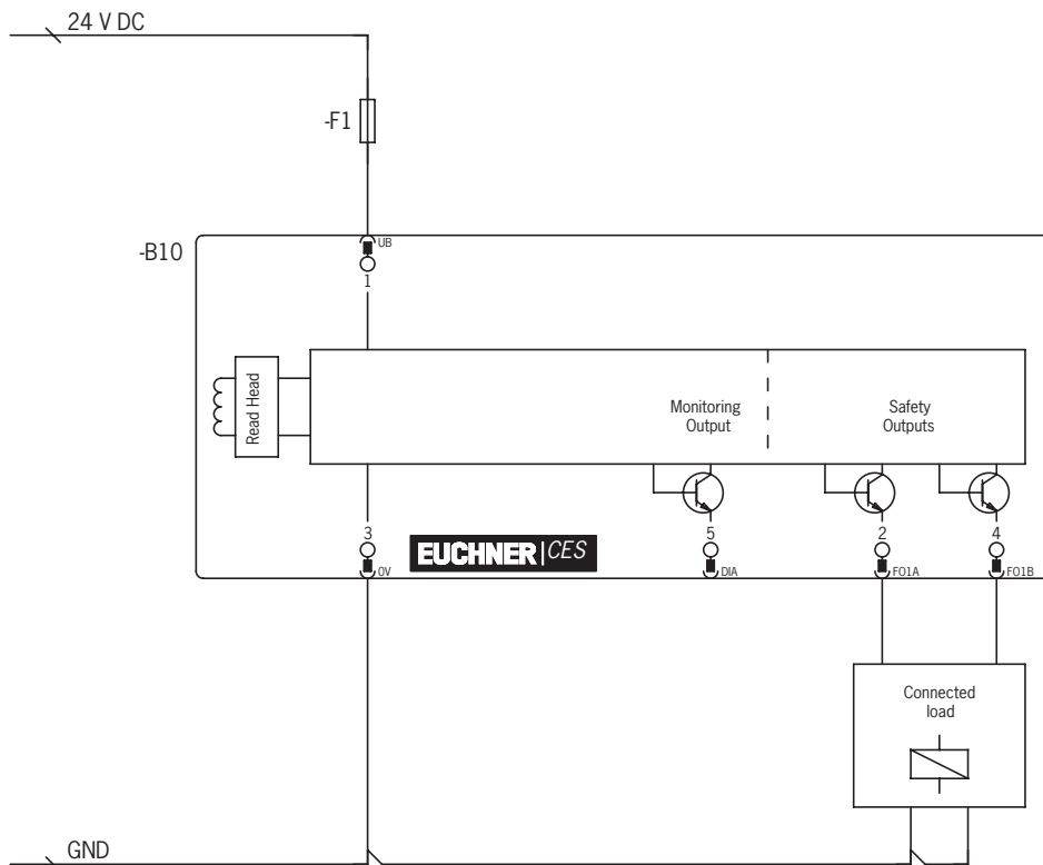
Obr. 2: Příklad připojení CES-I-AP-...
