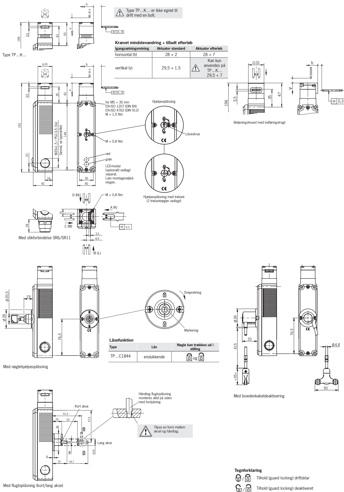
Figur 2: Måltægning TP...
