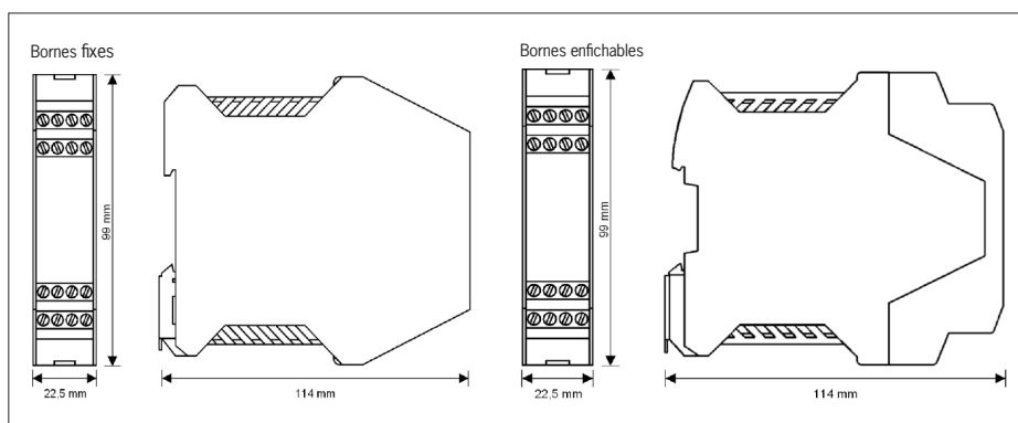
Fig. 4 : Dimensions ESM-BA2..
