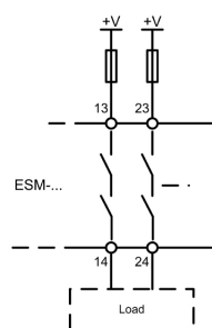
Fig. 16 : Raccordement des charges à commuter aux contacts de sécurité (exemple de configuration des contacts de sécurité. Peut être différente selon le type d'appareil. Tensions de commutation +V selon les caractéristiques techniques).
