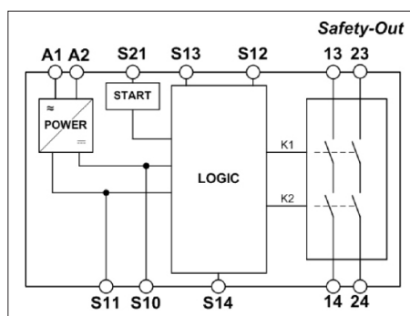
Fig. 1: Diagrama de bloques ESM-BA2..
