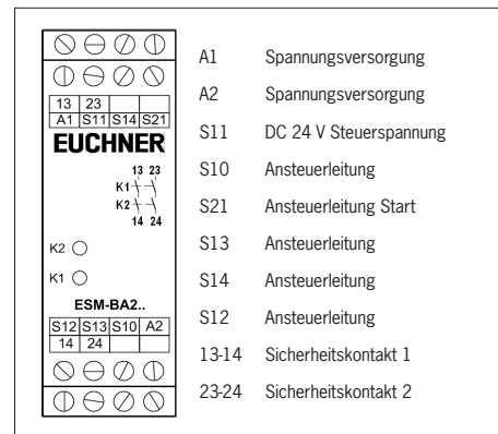
Bild 3: Anschlüsse
