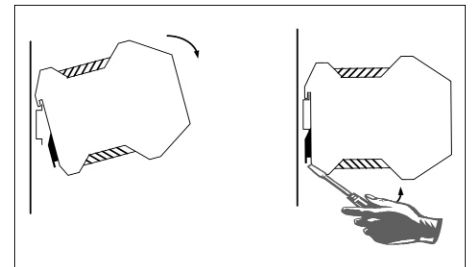
Fig. 2: Montaje/desmontaje
