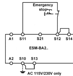
Fig. 7: Circuito de parada de emergencia monocanal con control de cortocircuitos a masa (categoría 1, hasta PL c).
