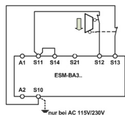
Bild 8: Zweikanalige Schiebeschutzgitter-Überwachung mit Querschuss- und Masseschluss-Überwachung (Kategorie 4, bis PL e).
