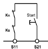
Bild 13: Rückführkreis. Überwachung extern angeschlossener Schütze oder Erweiterungsmodule.
