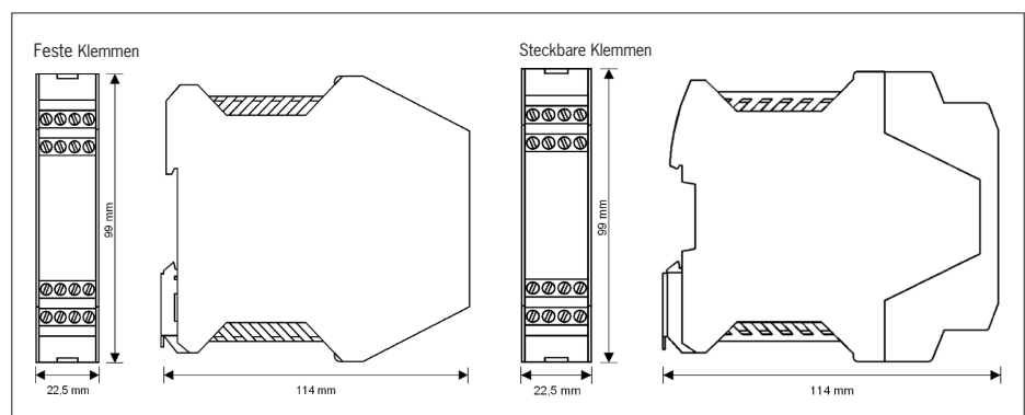
Bild 4: Maßzeichnung ESM-BA3..
