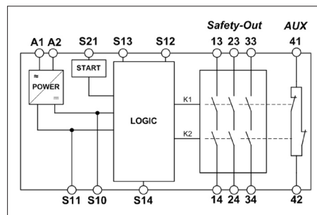
Bild 1: Blockschaubild ESM-BA3..
