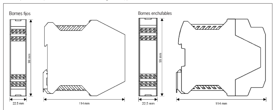
Fig. 4: Plano de dimensiones ESM-BA3..
