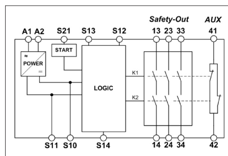
Bild 1: Blockschaltbild ESM-BA3..
