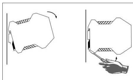
Fig. 2 : Montage / démontage
