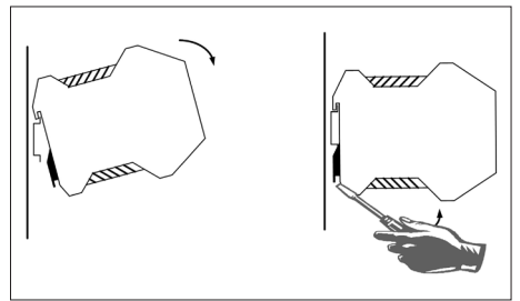
Bild 2: Montage/Demontage
