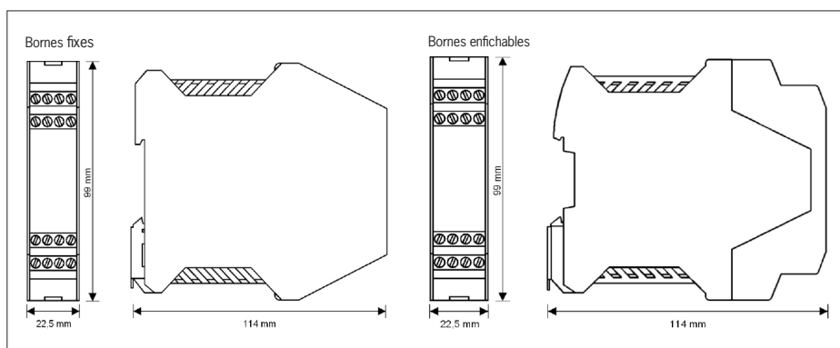
Fig. 4 : Dimensions ESM-BA3..
