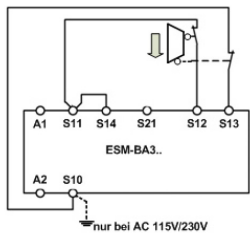
Bild 8: Zweikanalige Schiebenschutzgitter-Überwachung mit Querschuss- und Masseschluss-Überwachung (Kategorie 4, bis PL e).
