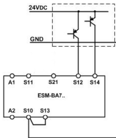
Bild 9: Zweikanalige Not-Halt-Schaltung mit pnp-Halbleiterausgängen/OSSD-Ausgängen mit Querschlosserkennung (Kategorie 4, bis PL e).
