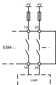
Fig. 16 : Raccordement des charges à commuter aux contacts de sécurité (exemple de configuration des contacts de sécurité. Peut être différente selon le type d'appareil. Tensions de commutation +V selon les caractéristiques techniques).
