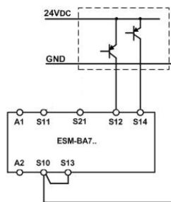
Fig. 9: Circuito de parada de emergencia de doble canal con salidas de semiconductor pnp/salidas OSSD con detección de errores de conexión cruzada (categoría 4, hasta PL e).
