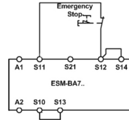
Fig. 7: Circuito de parada de emergencia monocanal con control de cortocircuitos a masa (categoría 1, hasta PL c).
