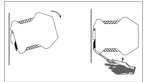
Bild 1: Montage/Demontage
