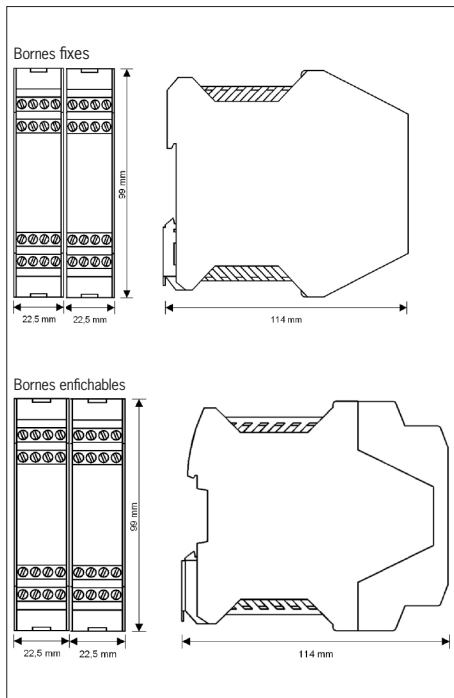
Fig. 2 : Dimensions ESM-BA7..
