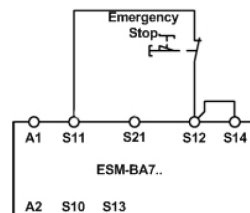
Fig. 7 : Circuit d'arrêt d'urgence monocanal avec détection des courts-circuits à la masse (catégorie 1, jusqu'à PL c).
