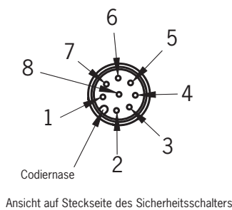
Bild 2: Steckerbelegung Sicherheitsschalter CES-AR-C01
