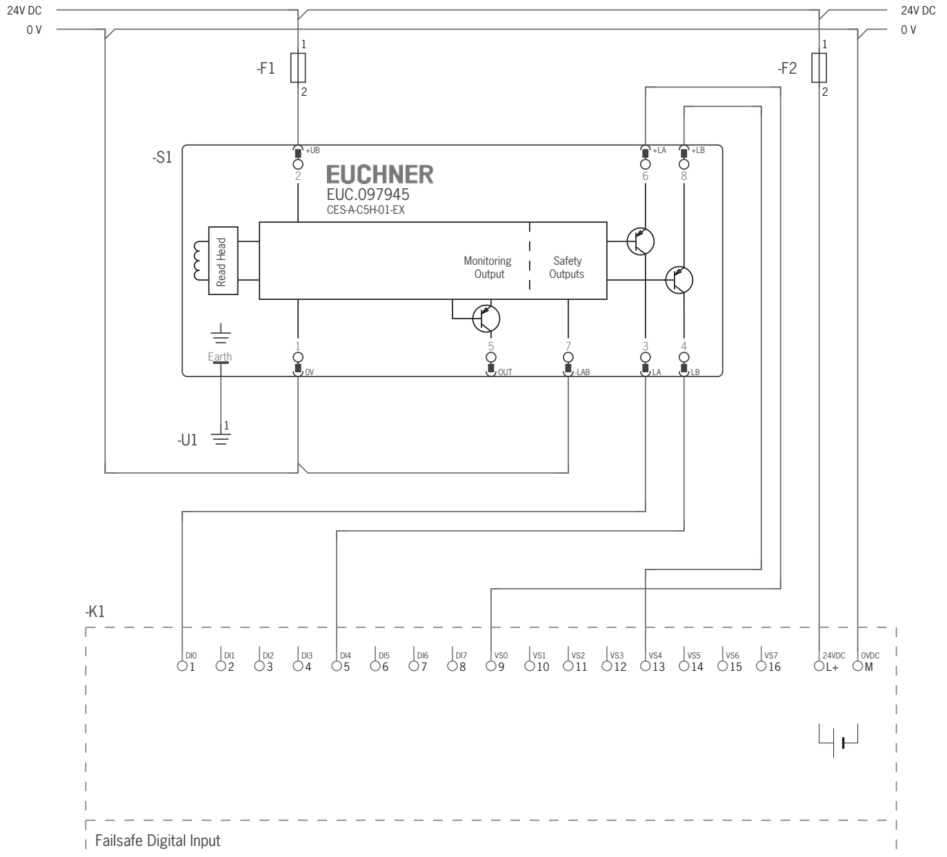
Bild 2: Anschlussbeispiel CES-A-C5H-01-EX
