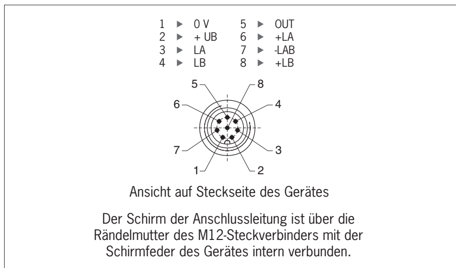
Bild 1: Steckerbelegung Sicherheitsschalter CES-A-C5H-01-EX
