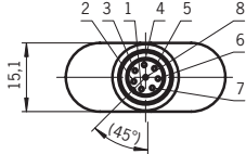
Buchse
