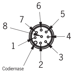
Ansicht auf Steckseite des Sicherheitsschalters
