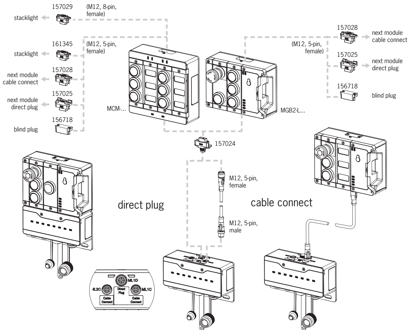
Bild 2: Module verbinden
