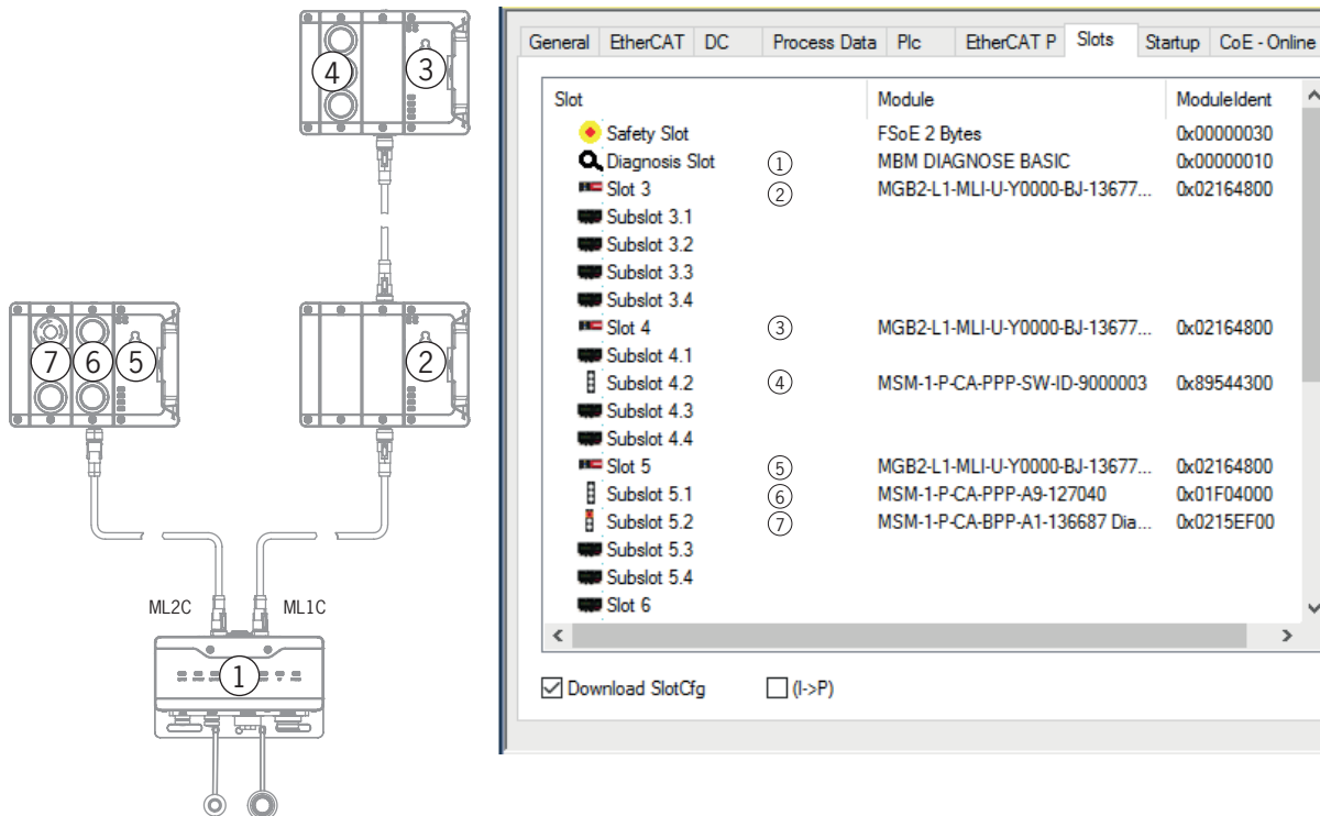
Bild 6: Beispielhaften Systemaufbau
