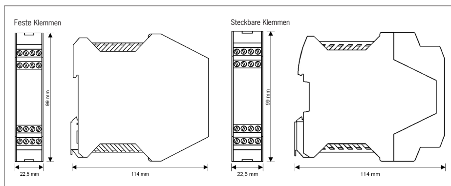
Bild 4: Maßzeichnung ESM-ES3..
