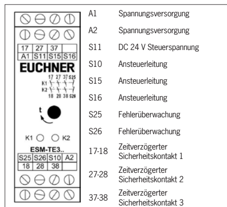
Bild 3: Anschlüsse
