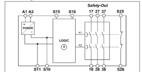
Bild 1: Blockschaltbild ESM-TE3..
