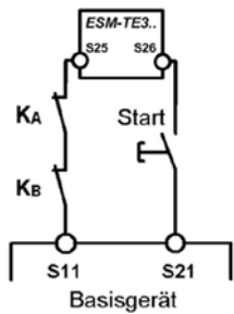
Bild 7: Rückführkreis mit überwachtem manuellen Start. Überwachung extern angeschlossener Schütze oder Erweiterungsmodule.
