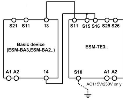
Fig. 5 : Raccordement ESM-TE3.. à l'unité de base
