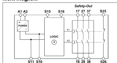
Bild 1: Blockschaltbild ESM-TE3..
