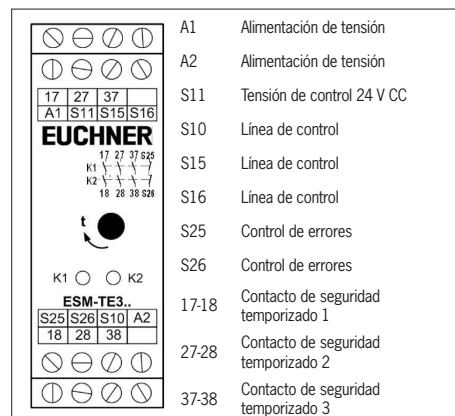
Fig. 3: Conexiones
