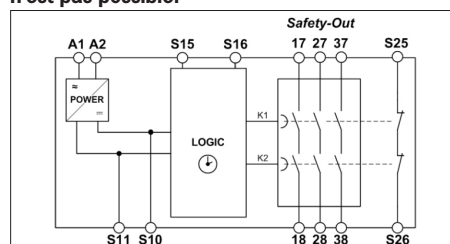
Fig. 1 : Schéma électrique ESM-TE3..
