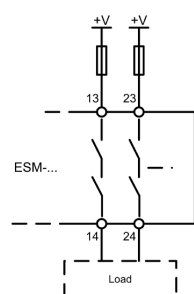
Fig. 10: Conexión de cargas conmutables a contactos de seguridad (ejemplo de configuración de los contactos; varía según el tipo de dispositivo; voltajes de conmutación +V según los datos técnicos).
