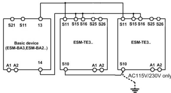
Fig. 6: Conexión de varios ESM-TE3.. al módulo básico.
