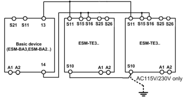
Fig. 6 : Raccordement de plusieurs ESM-TE3.. à l'unité de base
