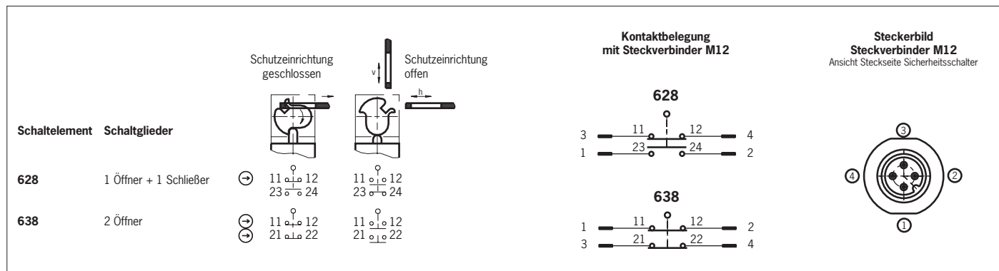
Bild 4: Schaltelemente und Schaltfunktionen
