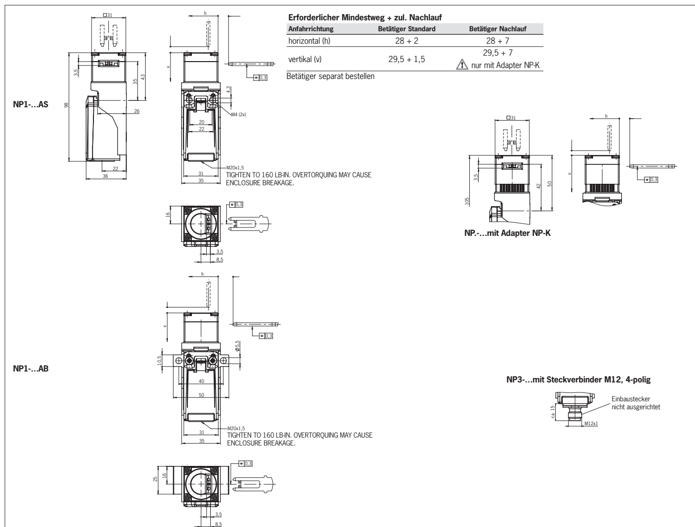
Bild 5: Maßzeichnung NP...
