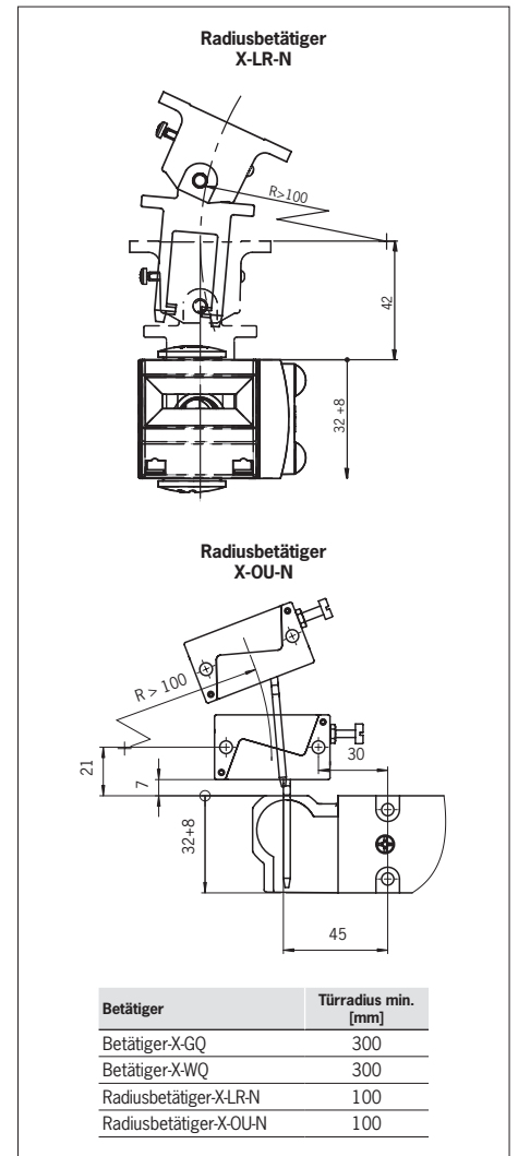
Bild 5: Minimale Türradien
