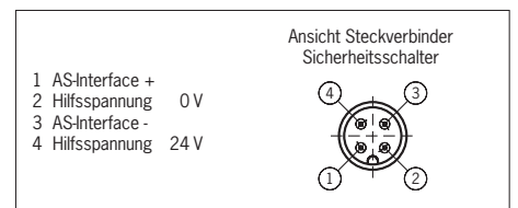
Bild 3: Anschlussbelegung M12-Steckverbinder
