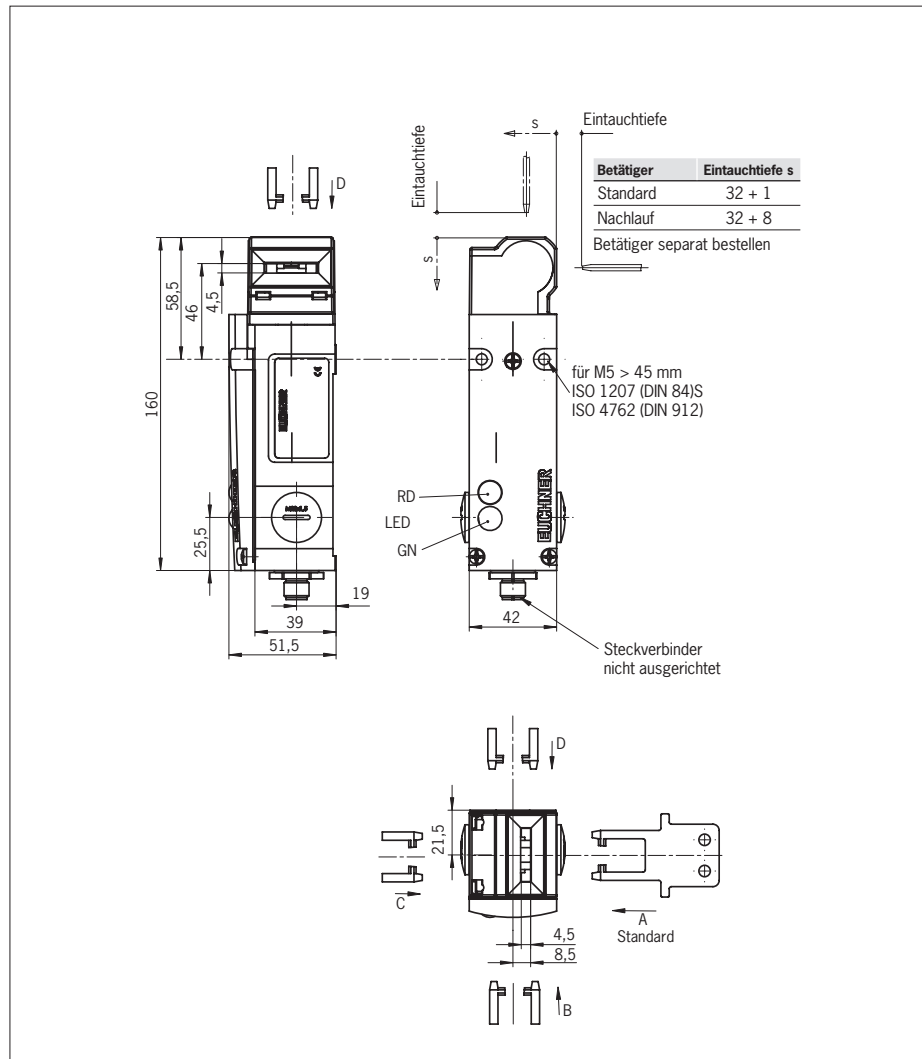
Bild 4: Maßzeichnung NX...AS
