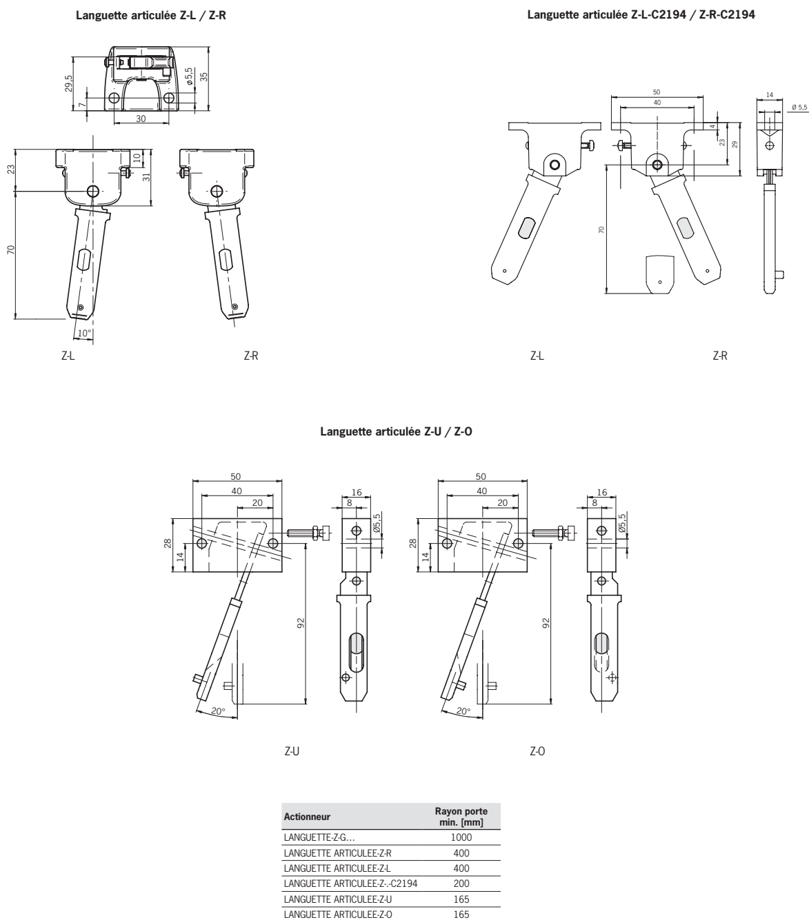
Fig. 10 : Rayons de porte minimum
