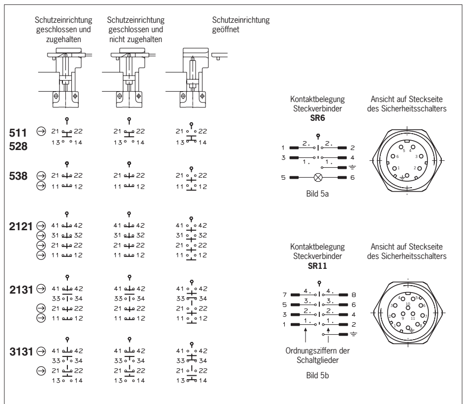
Bild 4: Schaltelemente mit Schaltfunktionen und Steckerbelegung
