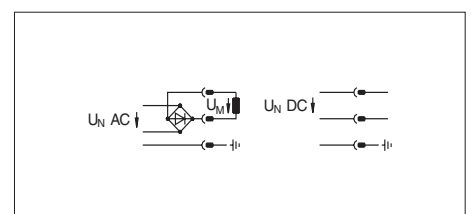
Bild 6: Steckverbinder für Magnetverriegelung
