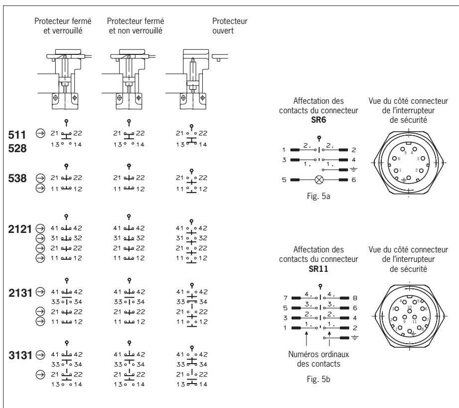
Fig. 4 : Éléments de commutation avec fonctions de commutation et affectation des broches
