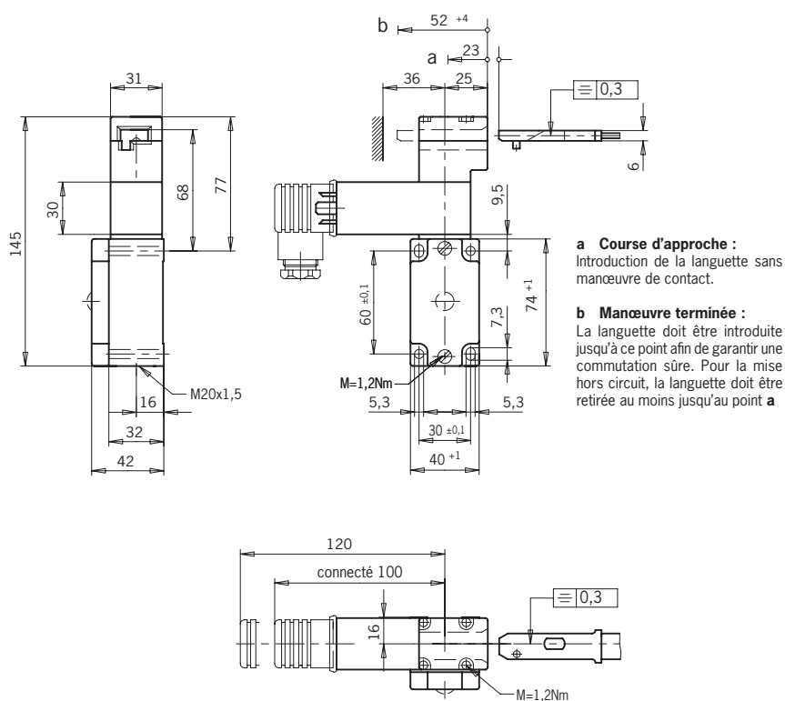
Fig. 7 : Dimensions NZ1VZ...VSM/VSE avec entrée de câble
