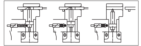
Fig. 1 : Type de verrouillage VSM
