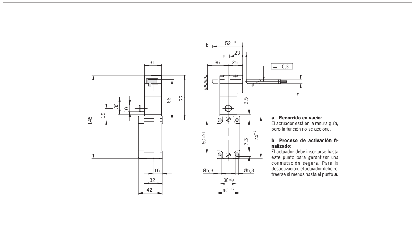
Fig. 8: Plano de dimensiones NZ1VZ...VSH con entrada de cable
