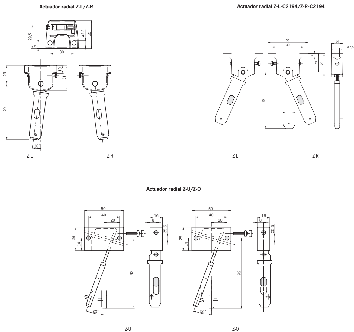
Fig. 11: Plano de dimensiones NZ2VZ-5... con conector SR11
