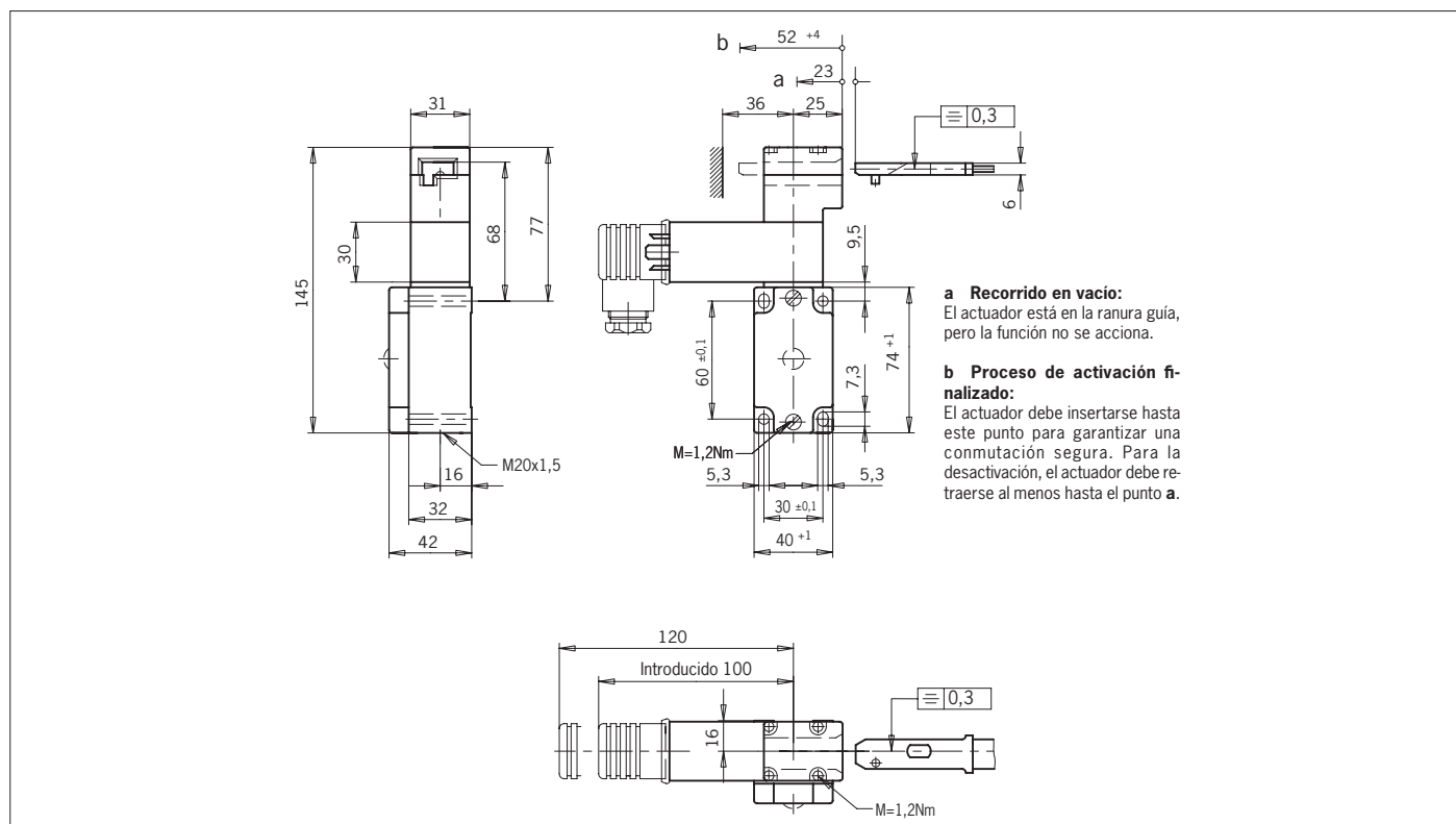
Fig. 7: Plano de dimensiones NZ1VZ...VSM/VSE con entrada de cable
