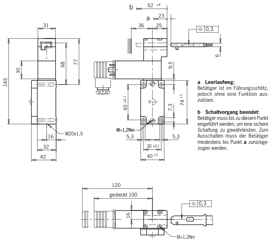
Bild 7: Maßzeichnung NZ1VZ-...VSM/VSE mit Leitungseinführung
