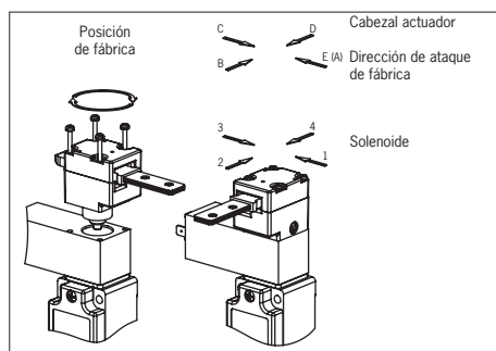
Fig. 3: Cambio de la dirección de accionamiento y de la posición del solenoide de bloqueo
