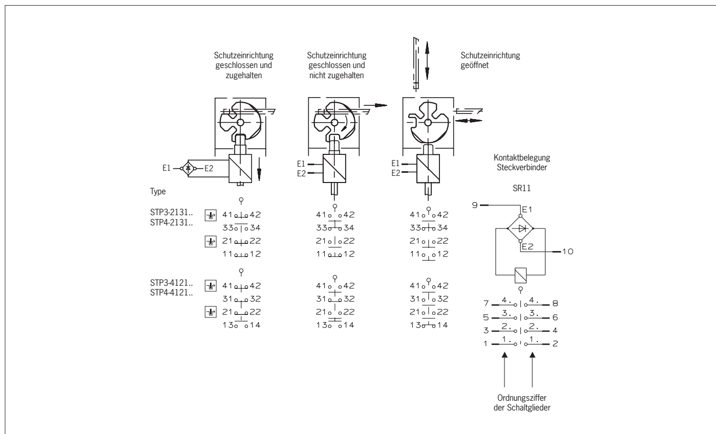
Bild 3: Schaltelemente und Schaltfunktionen
