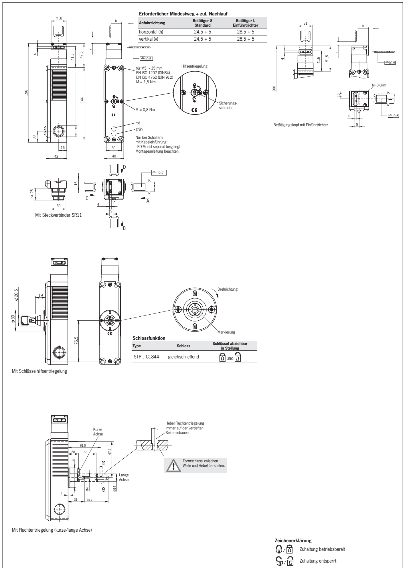
Bild 2: Maßzeichnung STP... ohne Einführtrichter und STP... mit Einführtrichter
