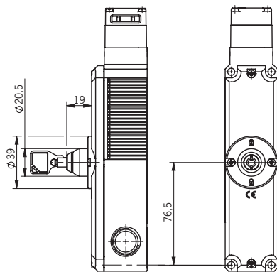
Mit Schlüsselhilfsentriegelung
