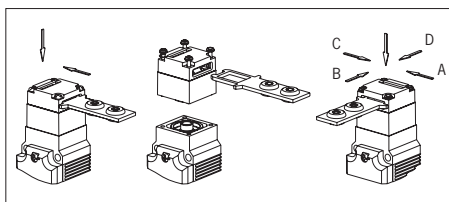
Fig. 1 : Changement de la direction d'actionnement
