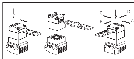
Bild 1: Umstellen der Betätigungsrichtung
