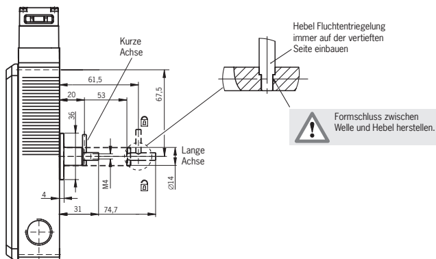
Mit Fluchentriegelung (kurze/ lange Achse)
