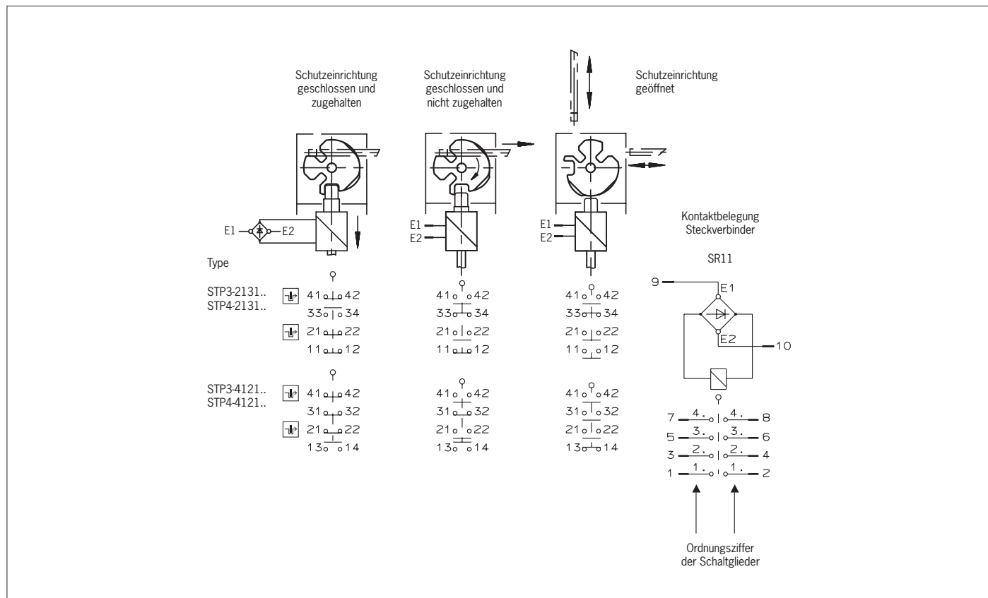
Bild 3: Schaltelemente und Schaltfunktionen
