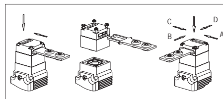
Fig. 1: Cambio de la dirección de accionamiento
