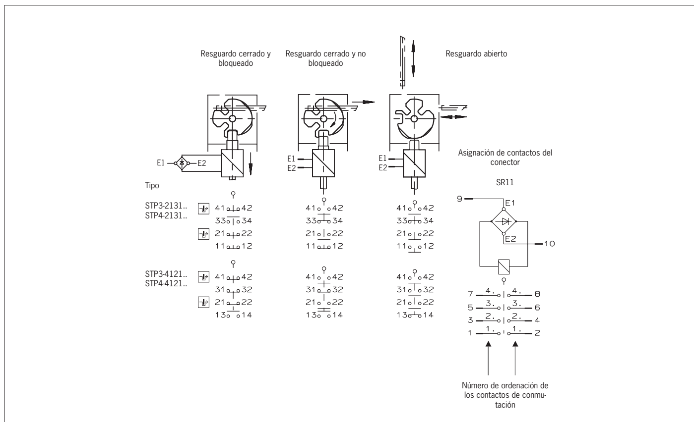
Fig. 3: Elementos interruptores y funciones de conmutación
