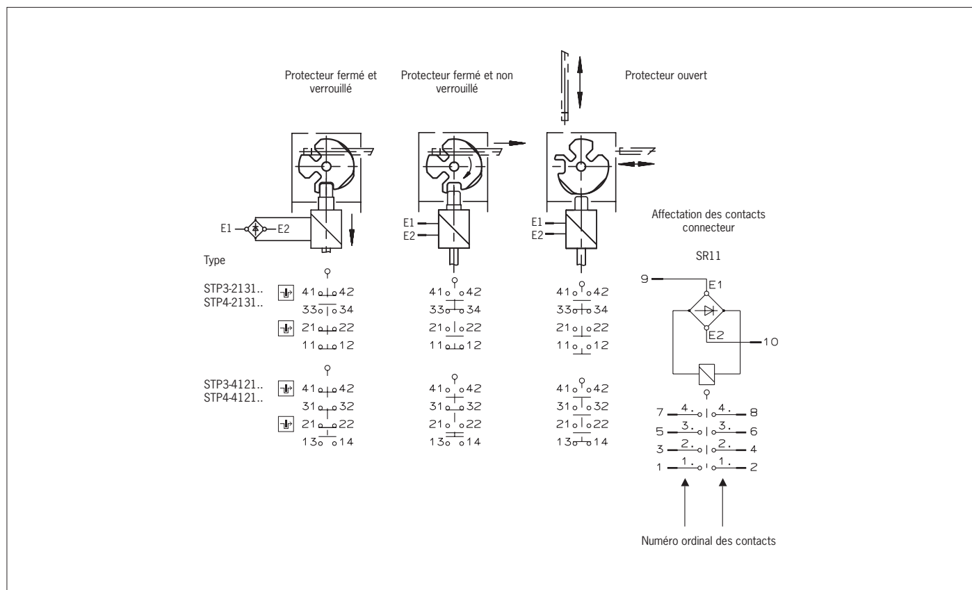
Fig. 3 : Éléments de commutation et fonctions de commutation
