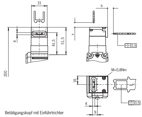
Betätigungs-kopf mit Einführtrichter
