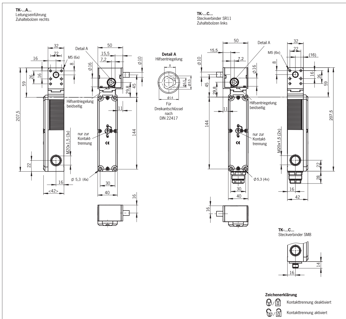
Bild 3: Maßzeichnung
