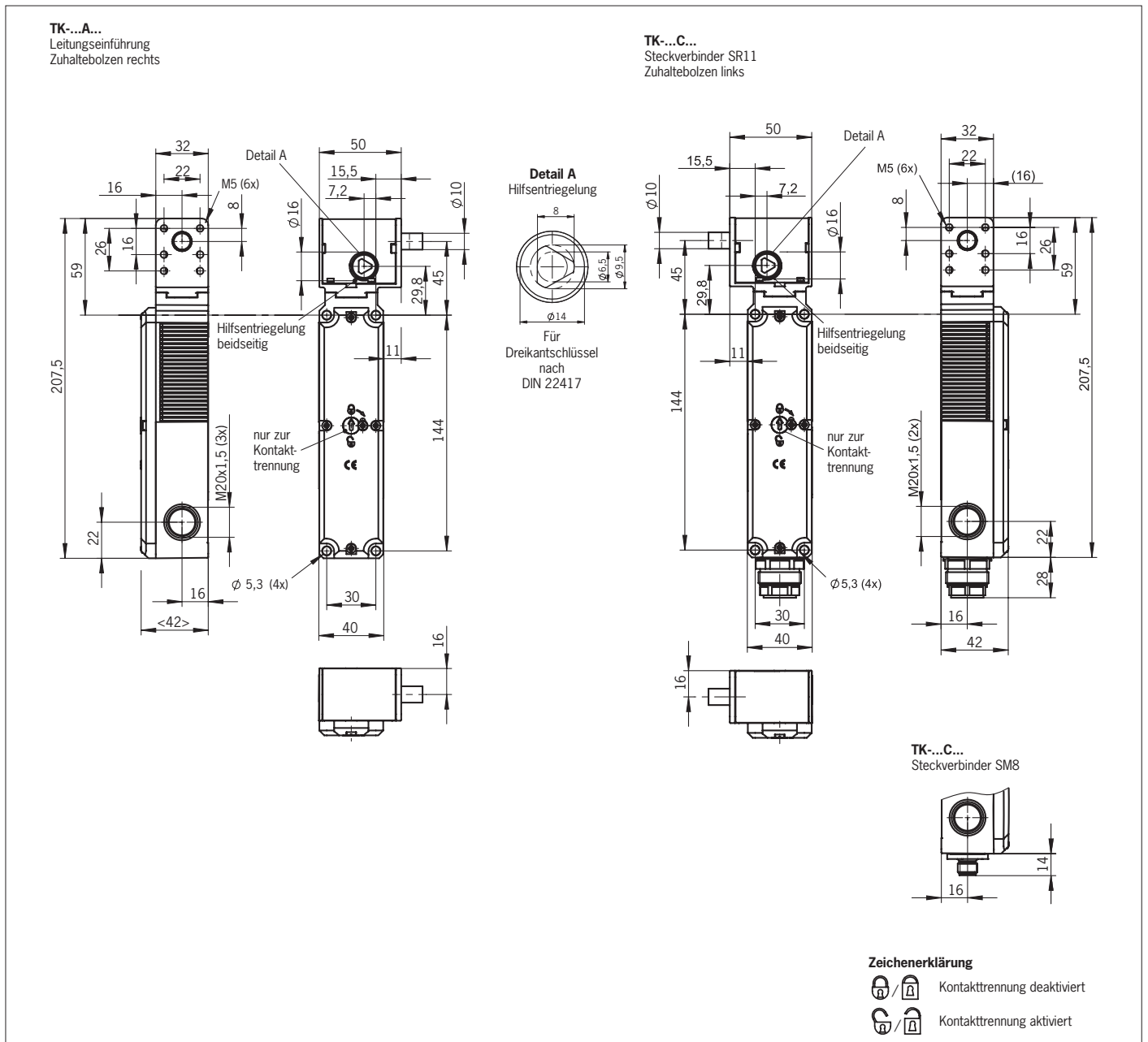
Bild 3: Maßzeichnung
