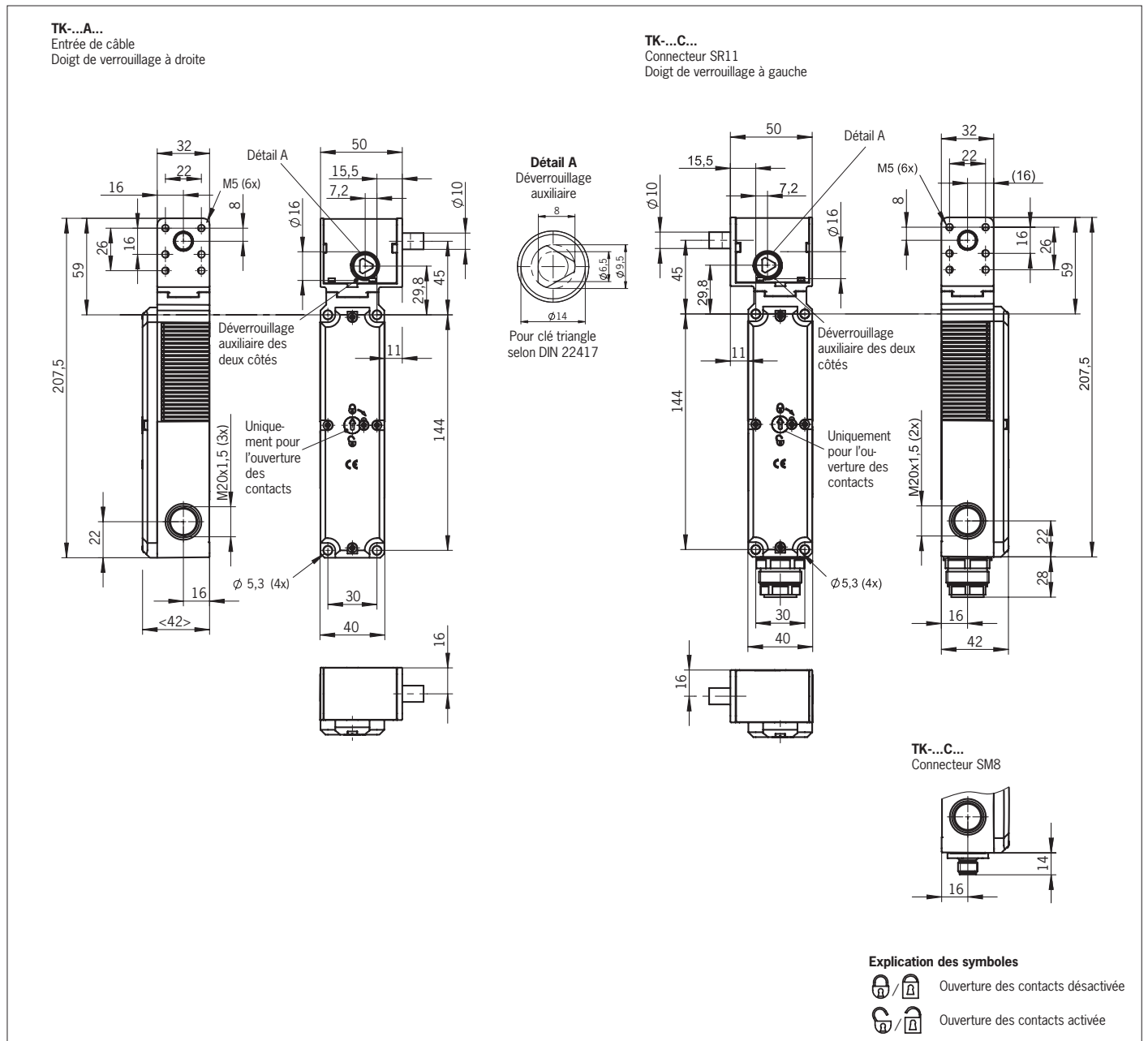
Fig. 3 : Dimensions
