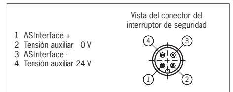
Fig. 3: Asignación de contactos del conector M12
