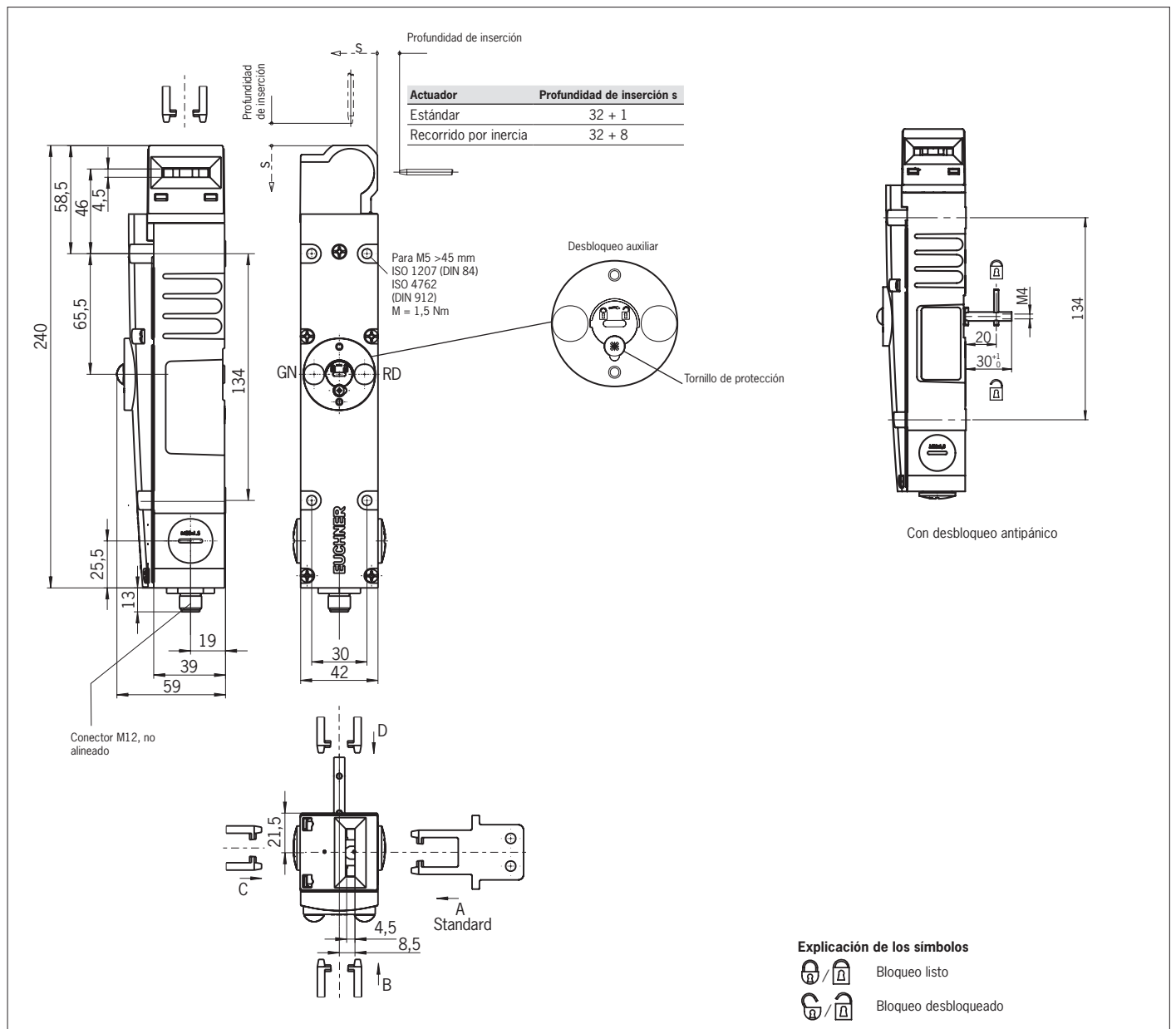
Fig. 4: Plano de dimensiones TX...AS1
