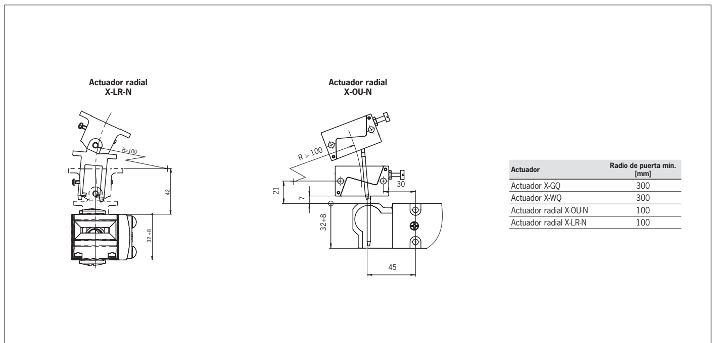
Fig. 5: Radios de puerta mínimos
