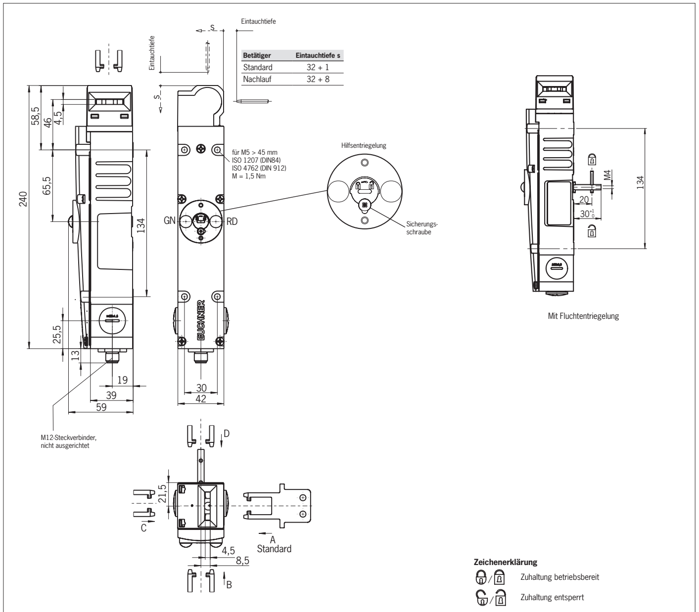
Bild 4: Maßzeichnung TX...AS1
