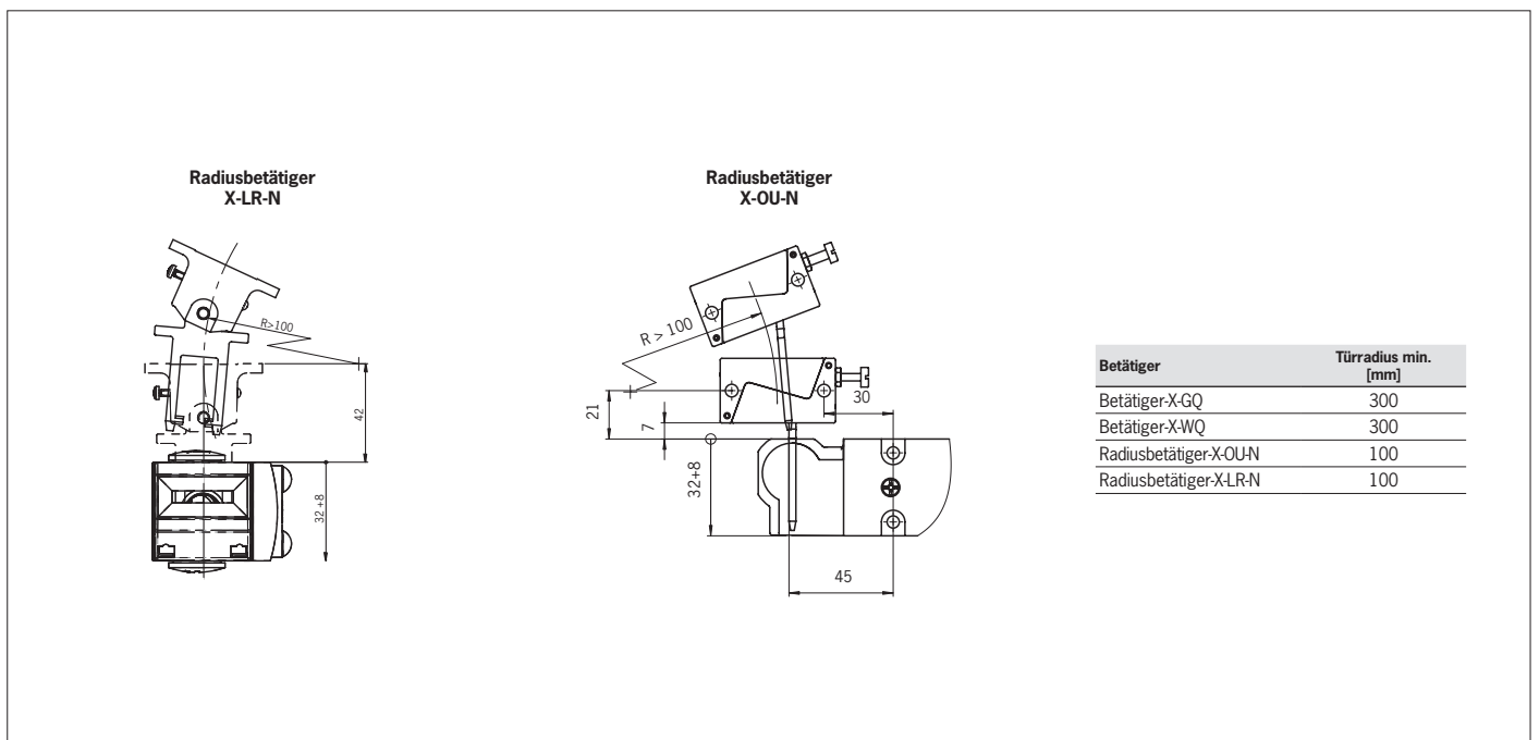
Bild 5: Minimale Türradien
