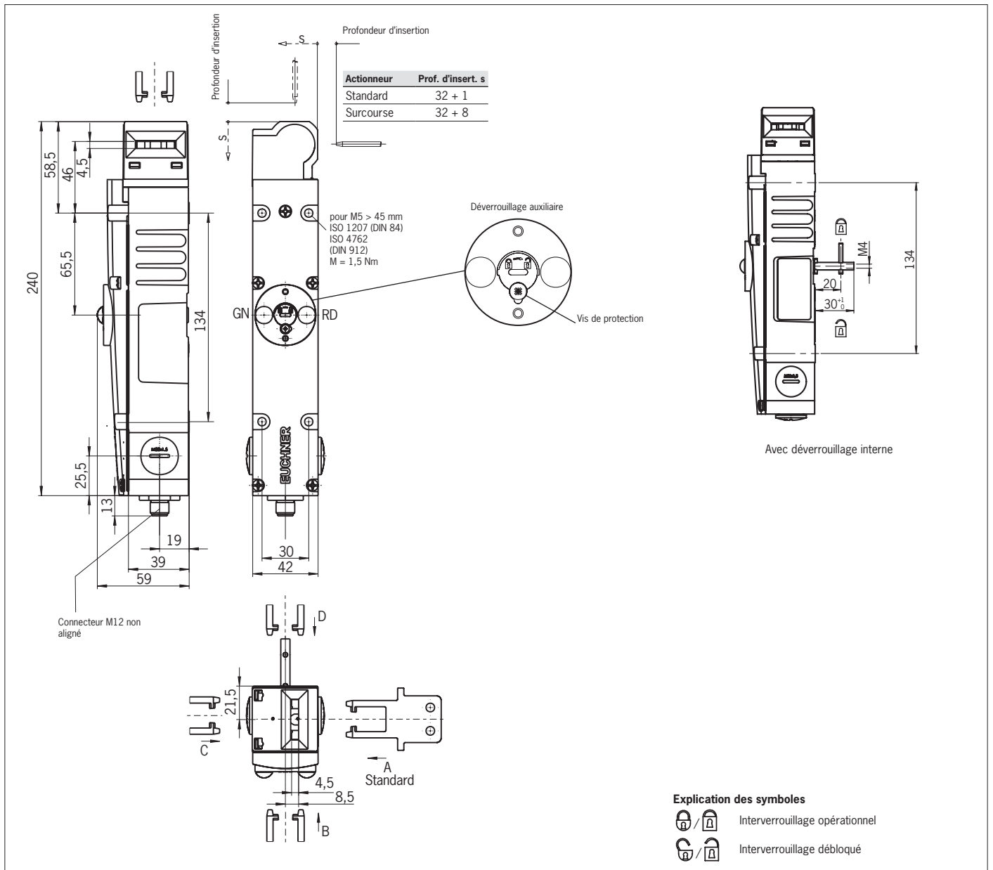
Fig. 4 : Dimensions TX...AS1
