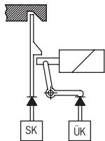
Schutzeinrichtung geschlossen und zugehalten
