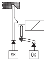
Schutzeinrichtung geschlossen und nicht zugehalten
