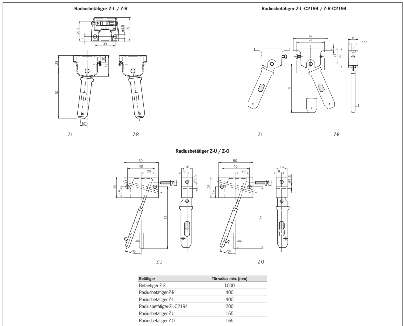
Bild 4: Minimale Türradien
