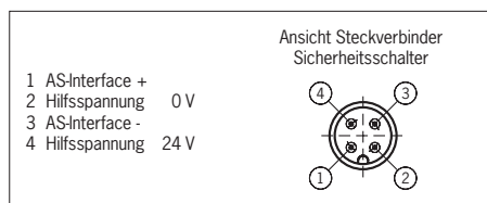
Bild 2: Anschlussbelegung M12-Steckverbinder
