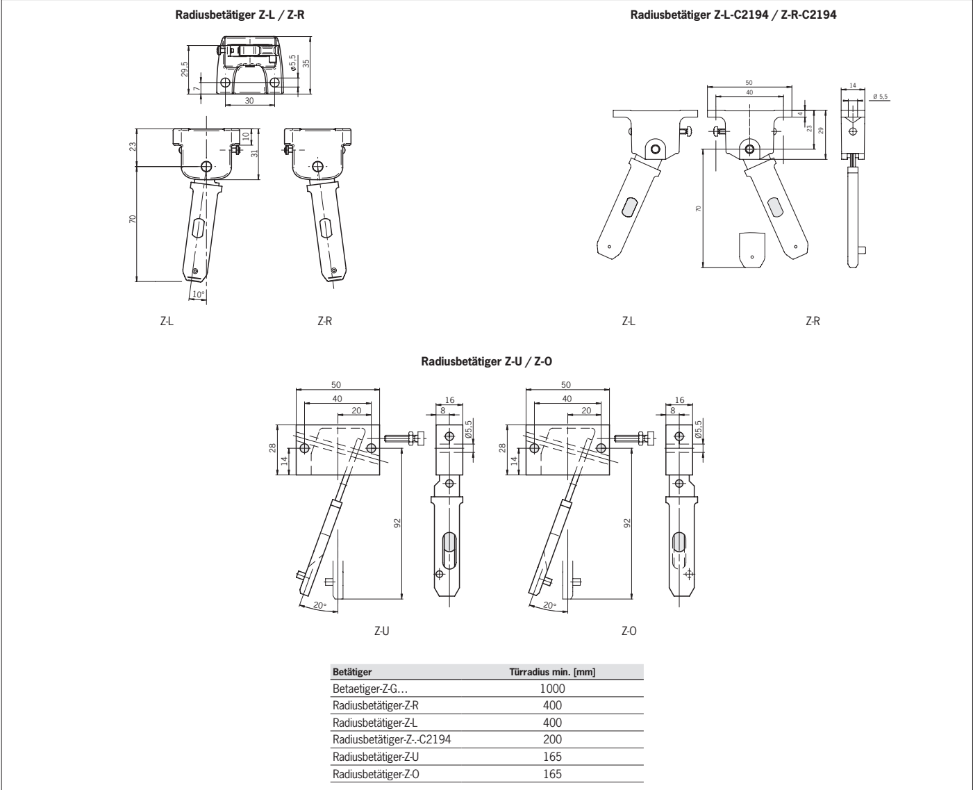
Bild 10: Minimale Türradien
