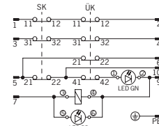
TZ..BHA...C1903/C2148/C2399 (avec connecteur BHA12)
