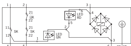
TZ..C1527 (con cable de conexión)
