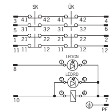
TZ..BHA...RC2408 (mit Steckverbinder BHA12)
