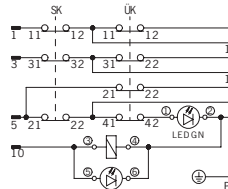
TZ..BHA...C1902 (avec connecteur BHA12)
