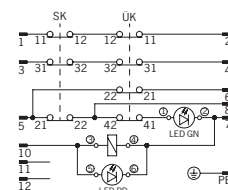
TZ..BHA...RC1924 (mit Steckverbinder BHA12)
