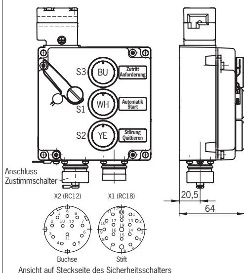
Bild 8: TZ..VAB-C2189/2198 mit Leuchten/beleuchteten Tasten und Zustimmschalteranschluss
