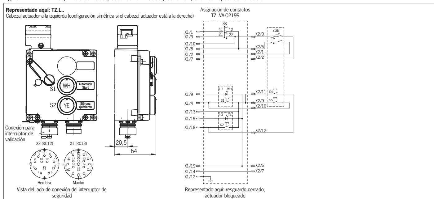
Fig. 9: TZ..VA-C2199 con botones iluminados y conexión para interruptor de validación
