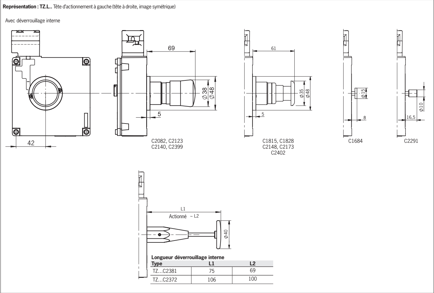
Fig. 4 : Dimensions déverrouillage interne
