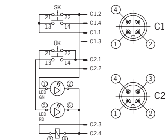
TZ..SEM4-C1888 (con conector 2 x M12, según DESINA)
