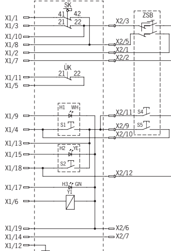
Bild 8: TZ..VAB-C2189/2198 mit Leuchten/beleuchteten Tasten und Zustimmschalteranschluss
