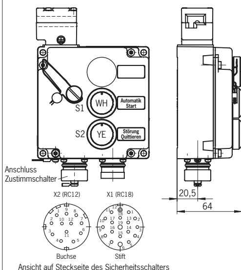
Bild 9: TZ..VA-C2199 mit beleuchteten Tasten und Zustimmschalteranschluss
