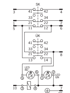
TZ..VABL12C-MF (avec connecteur BHA12)
