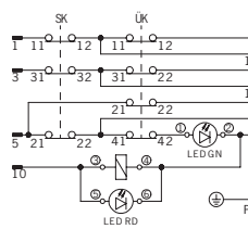
TZ..BHA...C1902 (mit Steckverbinder BHA12)
