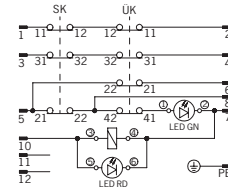
TZ..BHA...RC1924 (avec connecteur BHA12)
