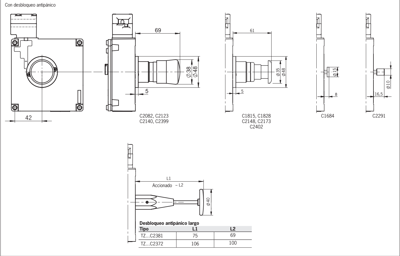
Fig. 4: Plano de dimensiones de los dispositivos de desbloqueo antipánico
