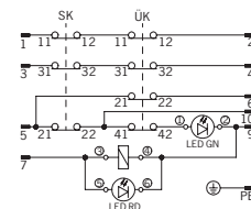
TZ..BHA...C1903/C2148/C2399 (mit Steckverbinder BHA12)
