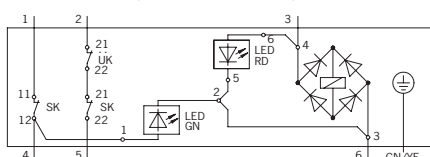
TZ..C1527 (mit Anschlussleitung)
