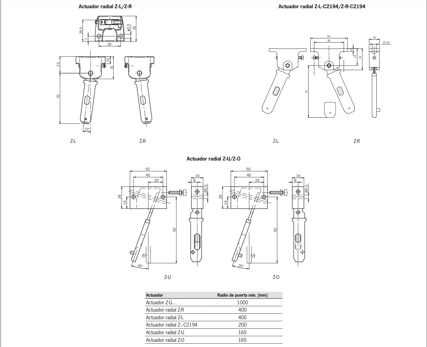
Fig. 10: Radios de puerta mínimos
