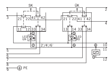
TZ..BHA...C1781 (mit Steckverbinder BHA12)
