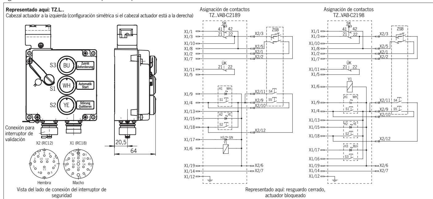
Fig. 8: TZ..VAB-C2189/2198 con luces/botones iluminados y conexión para interruptor de validación
