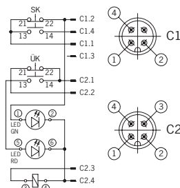
TZ..SEM4-C1888 (mit Steckverbinder 2 x M12, nach DESINA)
