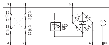
TZ...045177/045181/048492 (mit Steckverbinder SR6)
