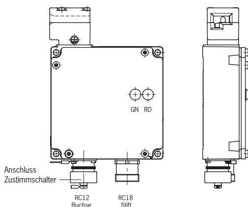
Bild 7: TZ..VAB-C1803 mit Zustimmschalteranschluss
