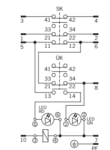
TZ..VABL12C-MF (mit Steckverbinder BHA12)
