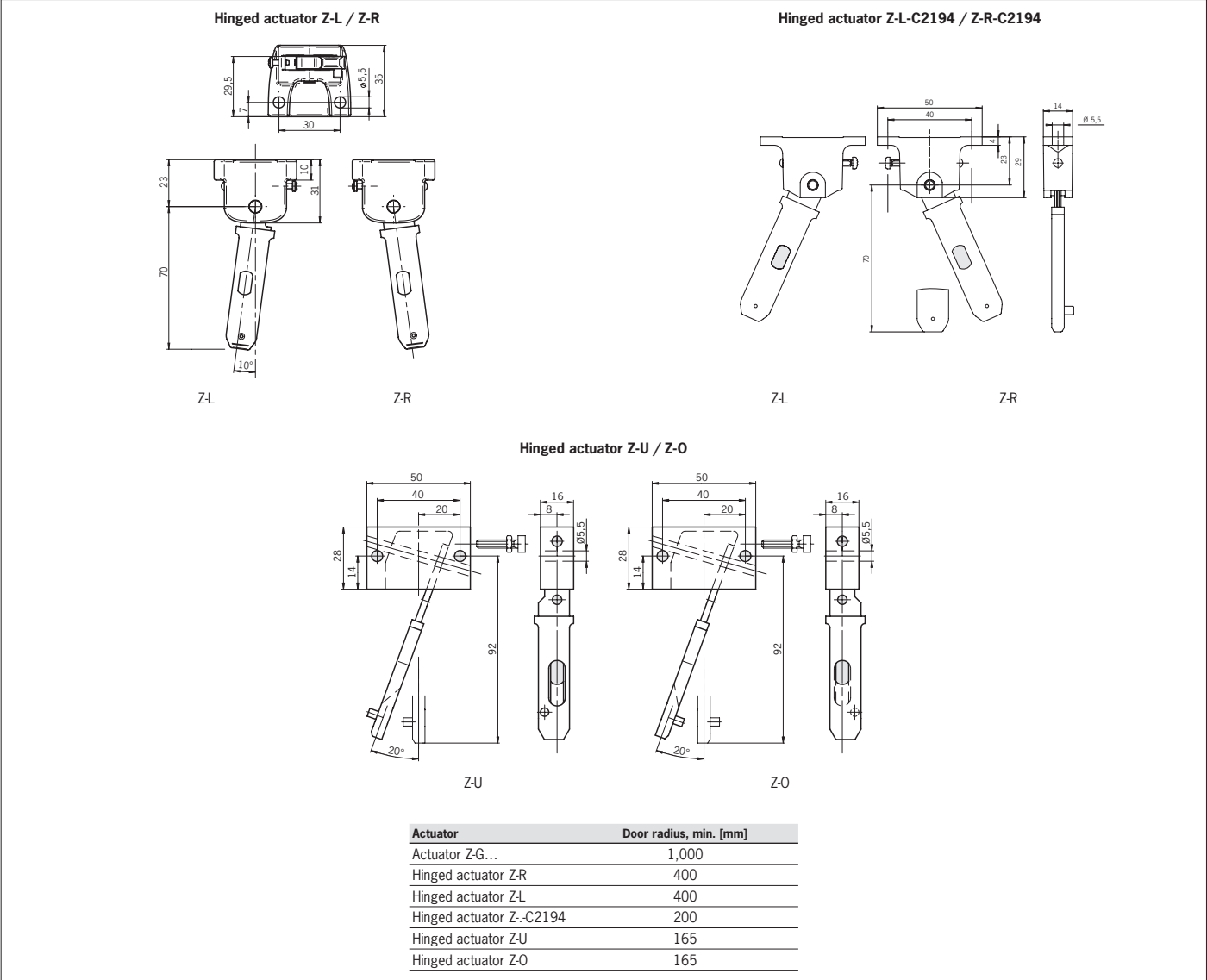
Fig. 10: Minimum door radii
