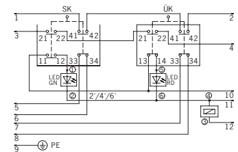
TZ..BHA...C1781 (avec connecteur BHA12)
