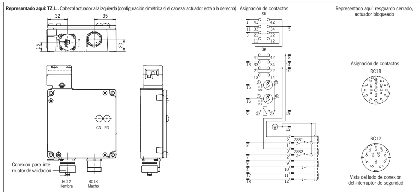
Fig. 7: TZ..VAB-C1803 con conexión para interruptor de validación
