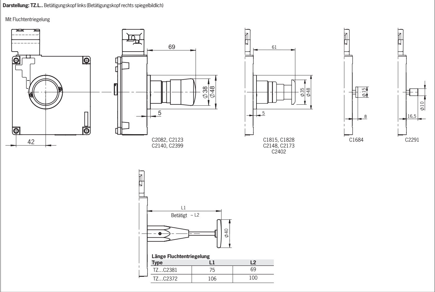
Bild 4: Maßzeichnungen Fluchtentriegelungen
