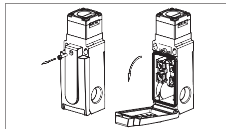
Fig. 2: Apertura del interruptor de seguridad
