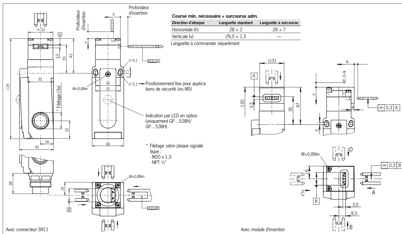
Fig. 4 : Dimensions GP...
