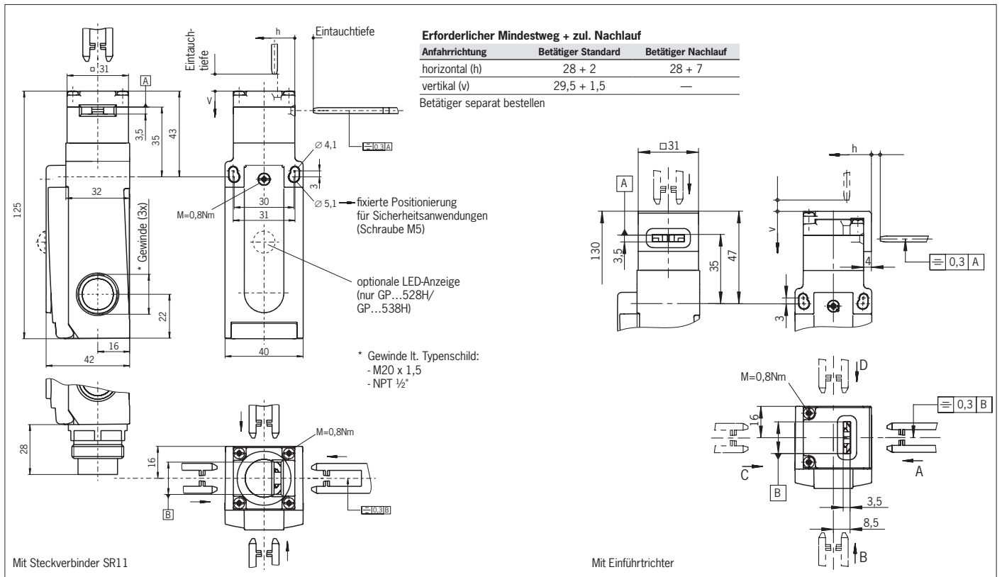
Bild 4: Maßzeichnung GP...
