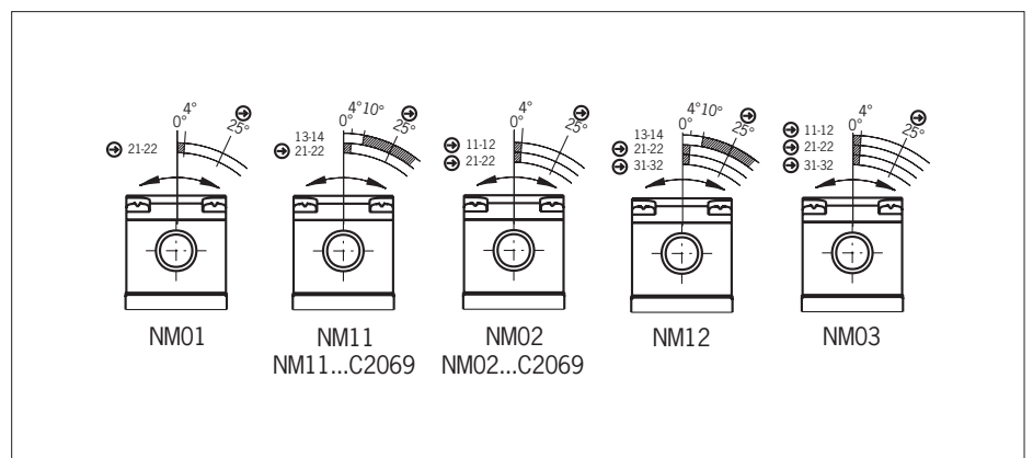
Fig. 4: Travel diagrams for NM..AK/NM..AG
