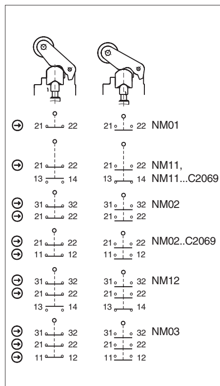
Bild 3: Schaltelemente und Schaltfunktionen
