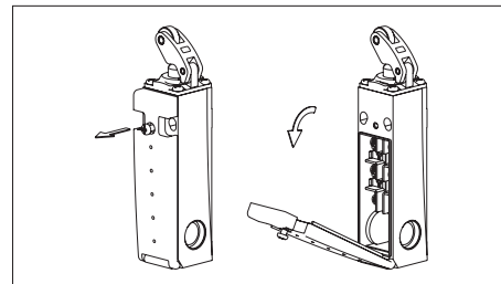
Bild 2: Öffnen des Sicherheitsschalters
