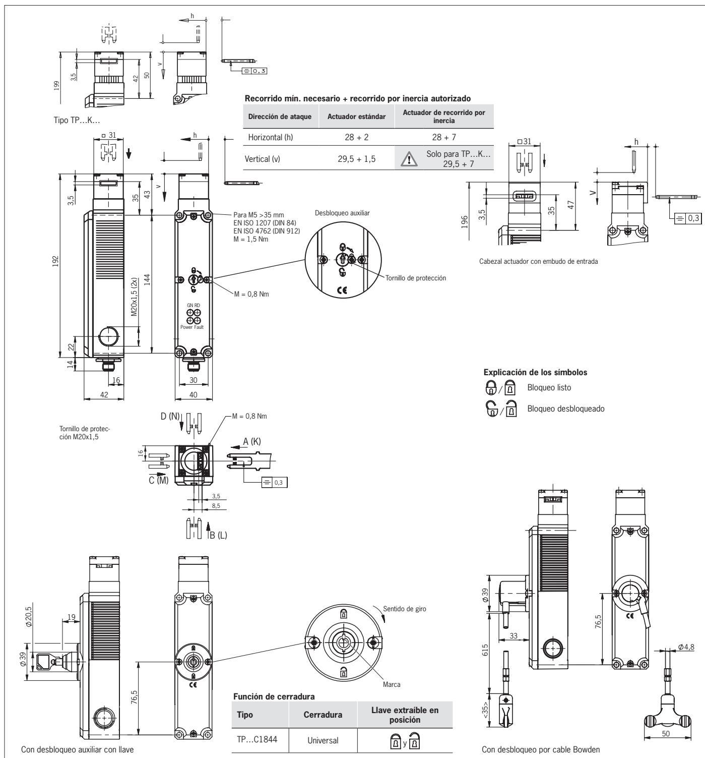
Fig. 3: Plano de dimensiones TP...AS2 sin embudo de entrada y TP...AS2 con embudo de entrada
