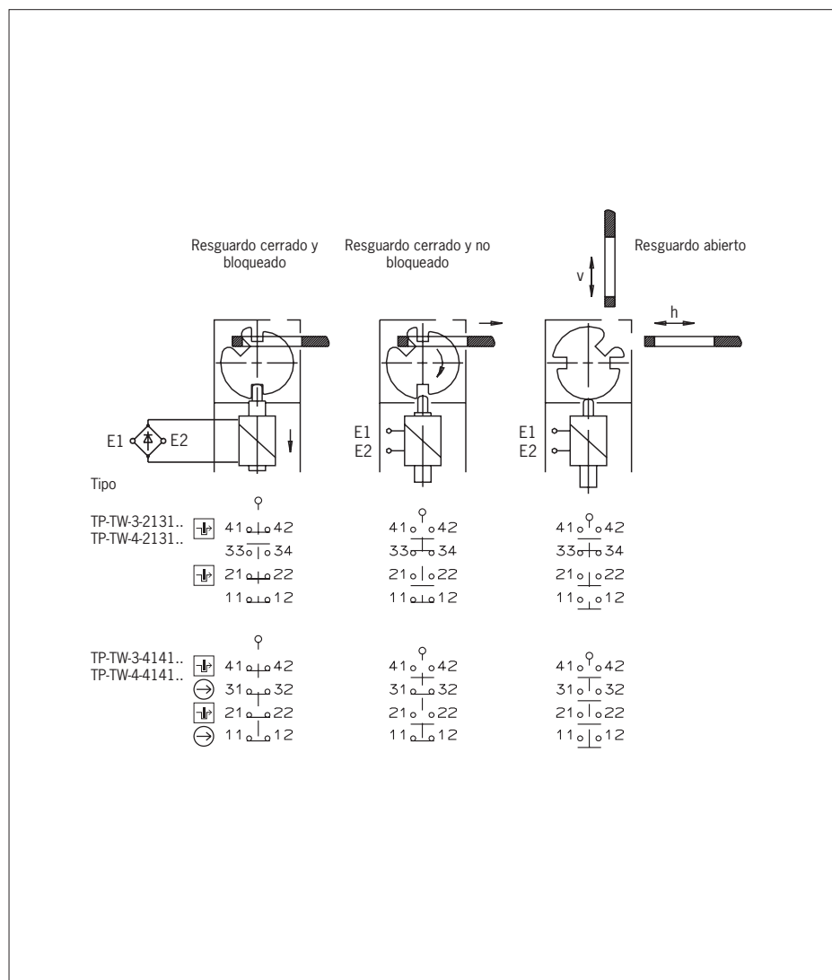
Fig. 4: Elementos interruptores y funciones de conmutación
