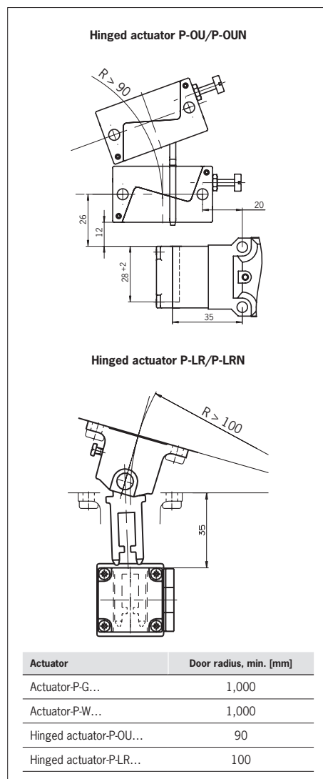
Fig. 5: Minimum door radii
