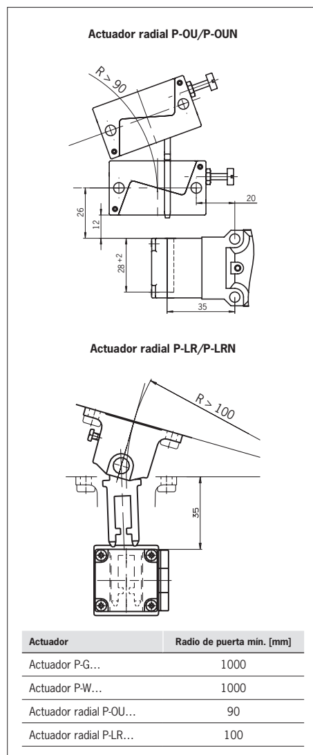
Fig. 5: Radios de puerta mínimos
