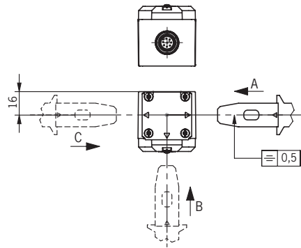
Cable outlet C
