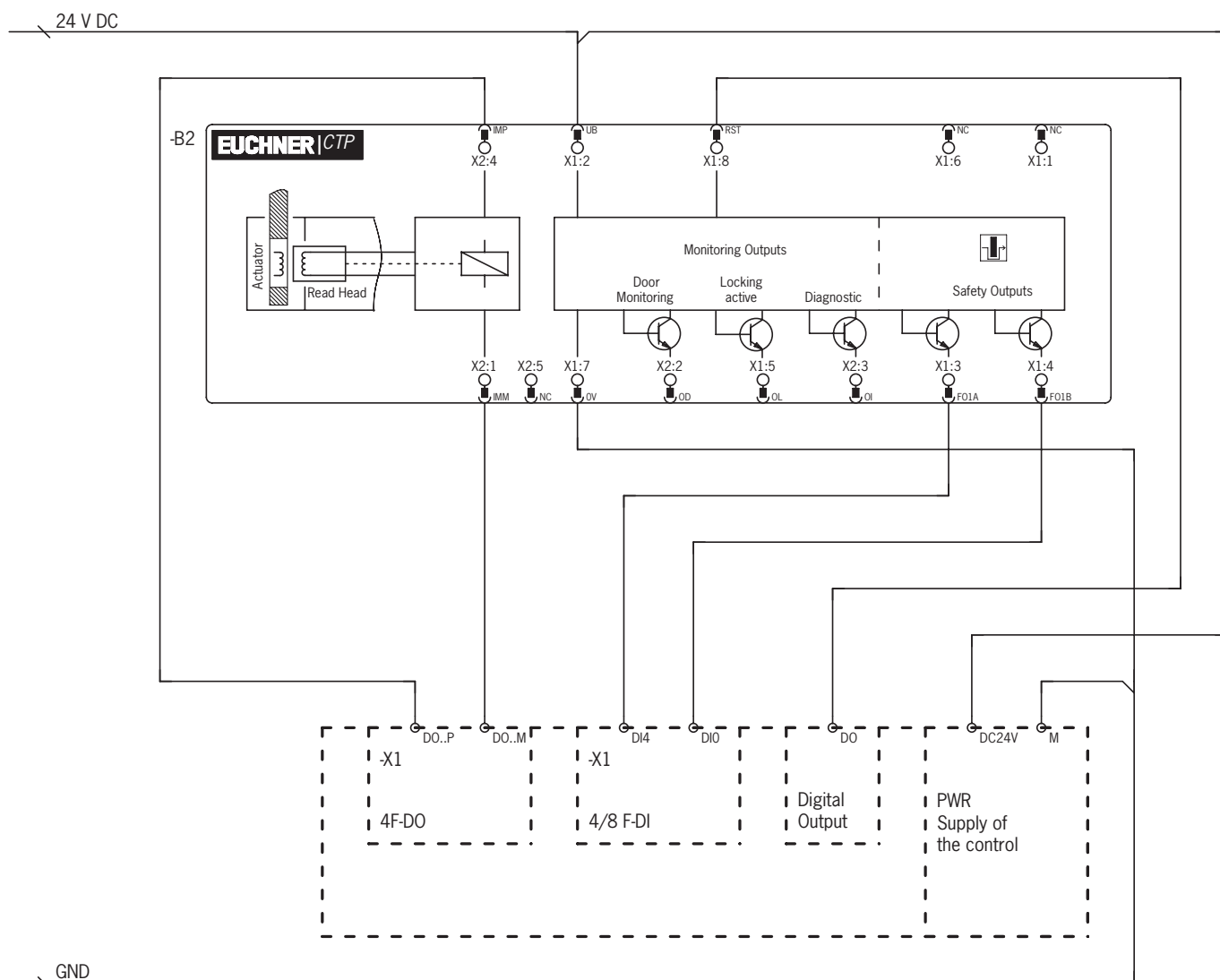
Figura 4: Ejemplo de conexión a ET200
