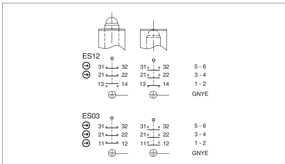
Fig. 2: Elementos interruptores y funciones de conmutación
