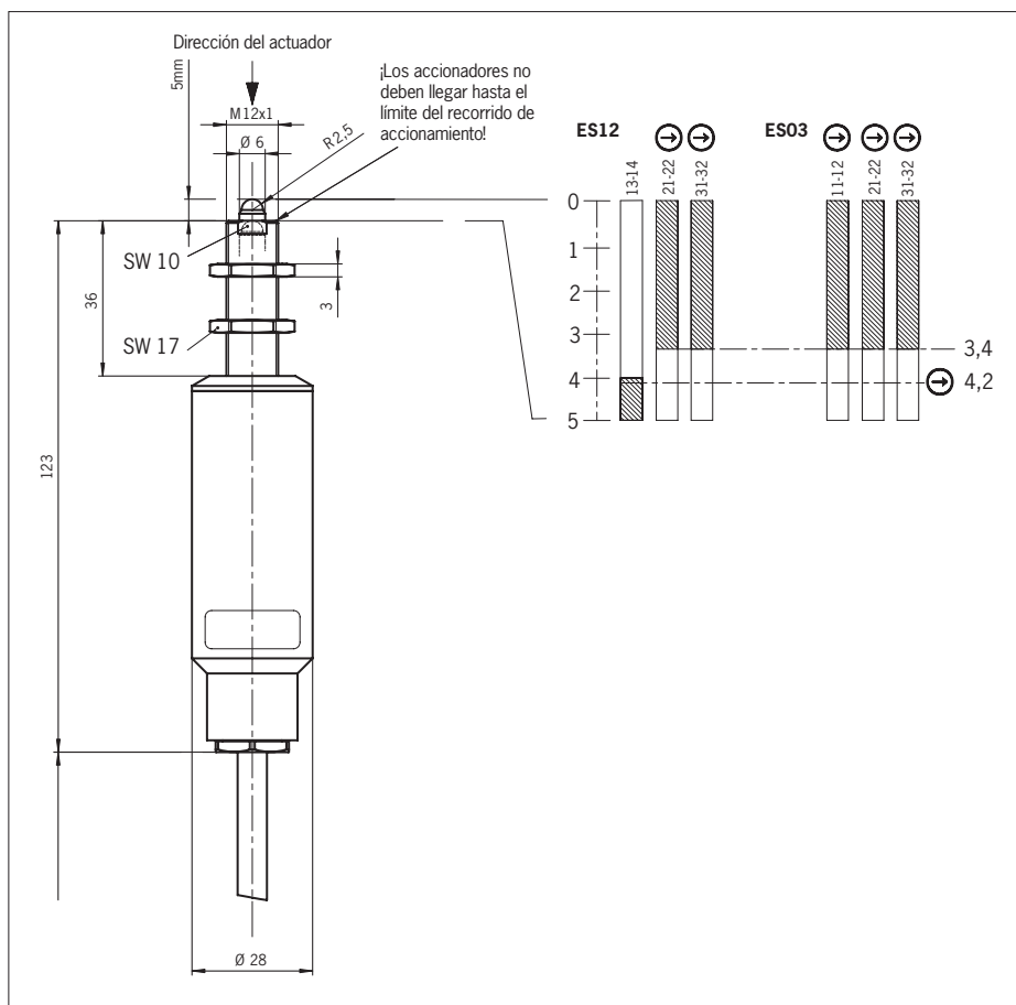
Fig. 1: Plano de dimensiones y diagramas de activación EGZ
