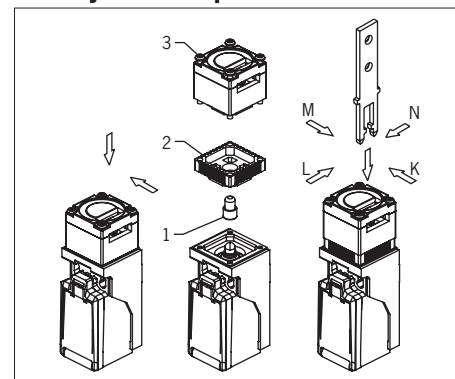
Fig. 2: Montaje del adaptador NP-K
