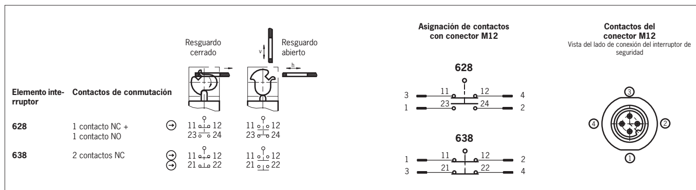
Fig. 4: Elementos interruptores y funciones de conmutación
