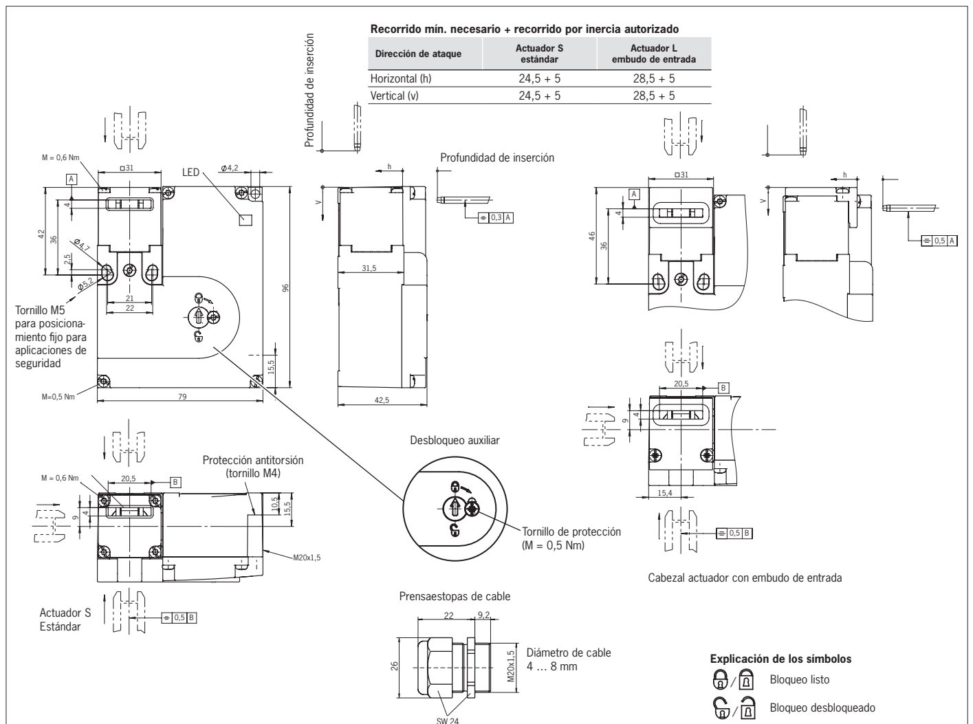
Fig. 6: Plano de dimensiones STM Pro sin embudo de entrada y STM Pro con embudo de entrada
