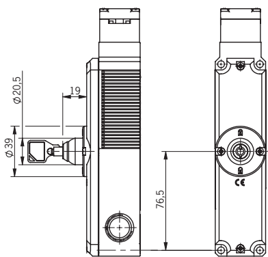
Con desbloqueo auxiliar con llave
