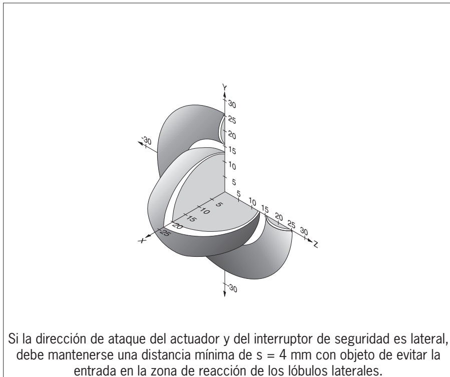
Fig. 6: Zona de reacción típica
