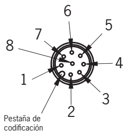
Vista del lado de conexión del interruptor de seguridad
