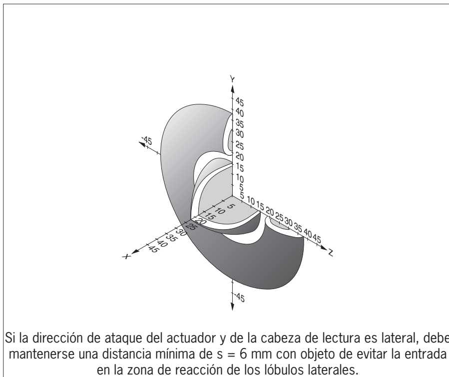
Fig. 8: Zona de reacción típica
