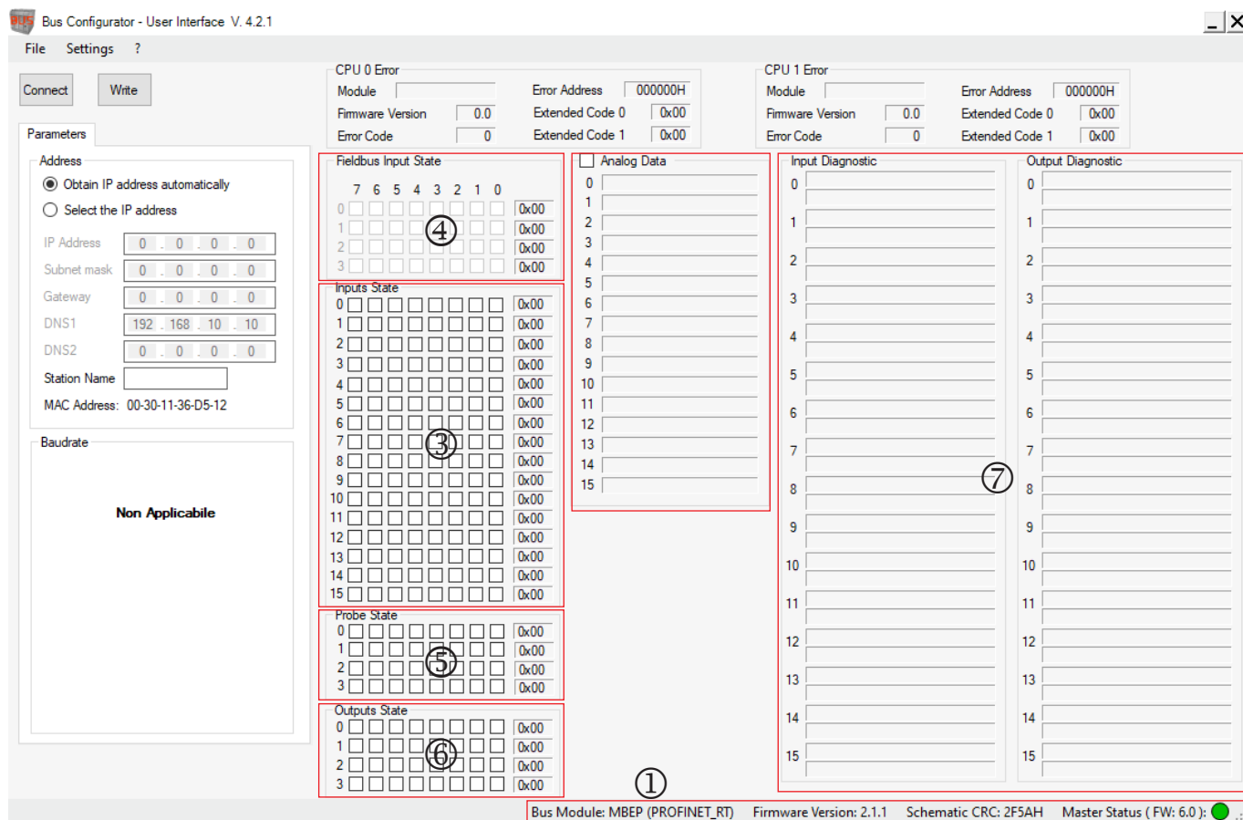
Fig. 6: Bus Configurator - User Interface, estructura de entrada y salida
