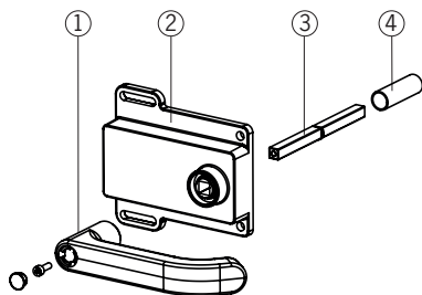
Fig. 4: Desbloqueo antipánico MGB-E-...
