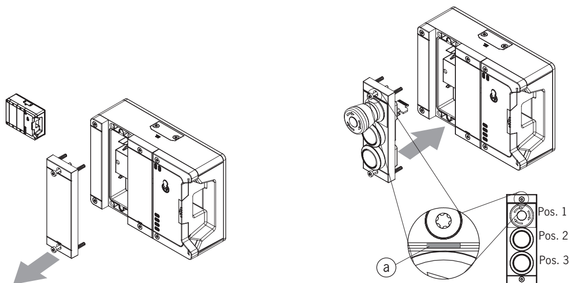
Fig. 10: Montaje de un submódulo
