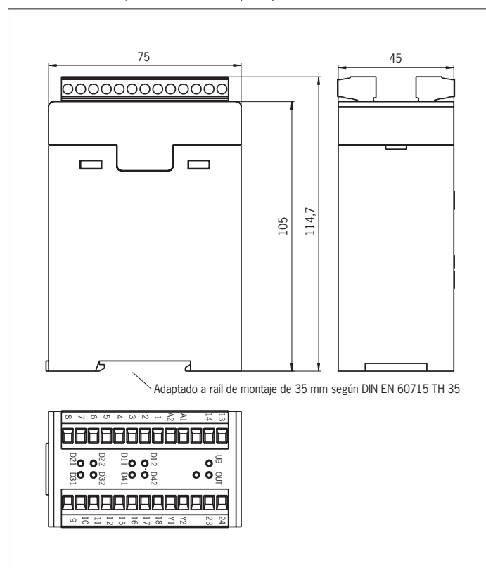
Fig. 1: Plano de dimensiones de la unidad de evaluación CMS-E-BR
