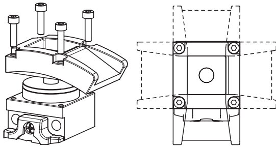
Fig. 1 : Changement de la direction d'attaque
