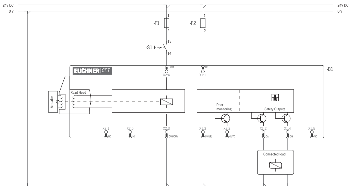
Fig. 5 : Repérage des bornes B, CET 3/4-AP avec 2 connecteurs M12, avec sortie d'état de porte Commande simple canal de l'électroaimant d'interverrouillage
