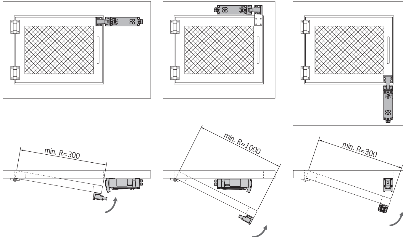
Fig. 2 : Emplacement de montage et rayons de porte
