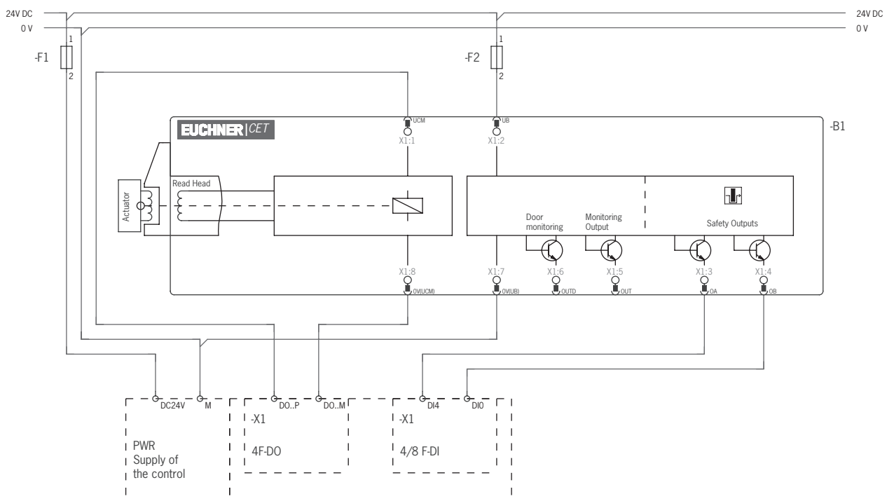
Fig. 8 : Repérage des bornes C/D, CET 3/4-AP avec 1 connecteur M12, avec sortie de signalisation OUT ou DIA sur X1:5 Commande double canal de l'électroaimant d'interverrouillage
