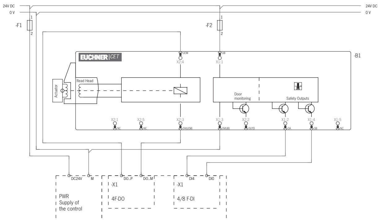
Fig. 6 : Repérage des bornes B, CET 3/4-AP avec 2 connecteurs M12, avec sortie d'état de porte Commande double canal de l'électroaimant d'interverrouillage
