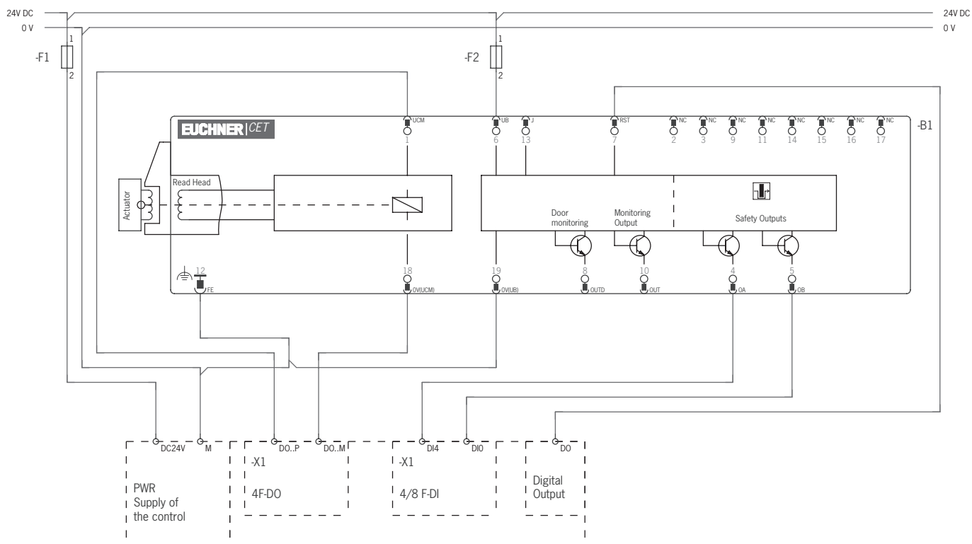
Fig. 10 : Repérage des bornes E, CET 3/4-AP avec 1 connecteur M23, Commande double canal de l'électroaimant d'interverrouillage
