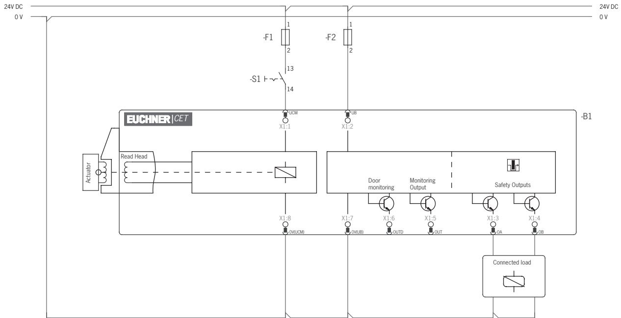
Fig. 7 : Repérage des bornes C/D, CET 3/4-AP avec 1 connecteur M12, avec sortie de signalisation OUT ou DIA sur X1:5 Commande simple canal de l'électroaimant d'interverrouillage
