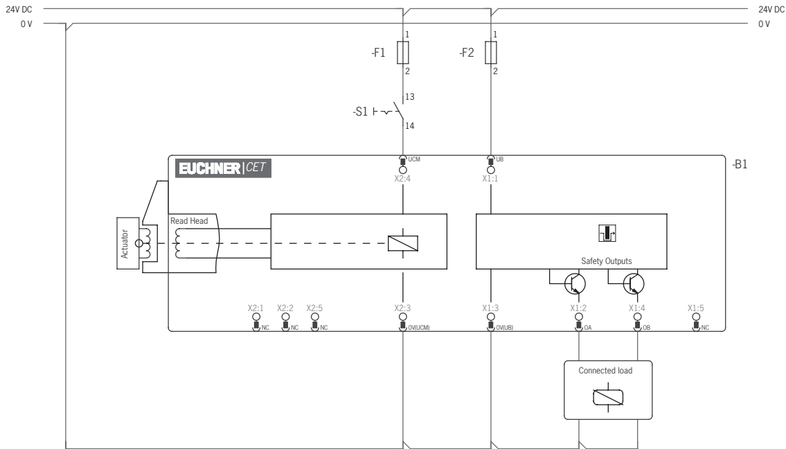
Fig. 3 : Repérage des bornes A, CET 3/4-AP avec 2 connecteurs M12, sans sortie d'état de porte Commande simple canal de l'électroaimant d'interverrouillage
