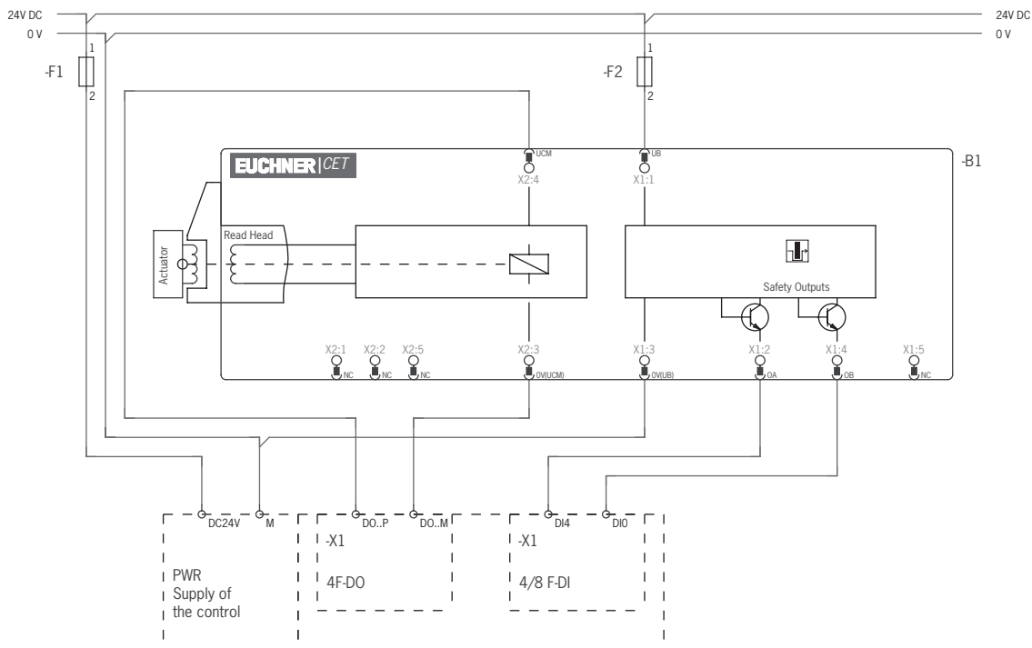
Fig. 4 : Repérage des bornes A, CET 3/4-AP avec 2 connecteurs M12, sans sortie d'état de porte Commande double canal de l'électroaimant d'interverrouillage
