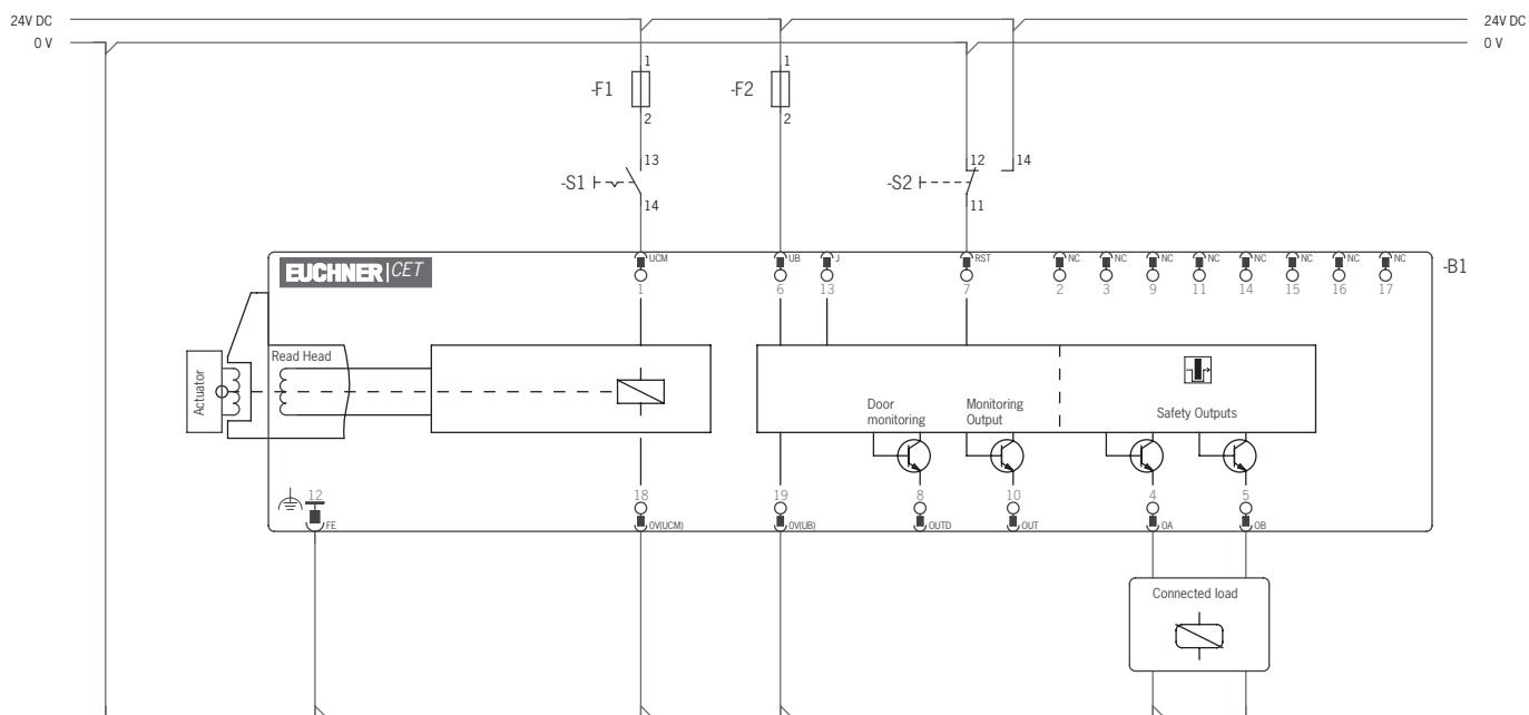
Fig. 9 : Repérage des bornes E, CET 3/4-AP avec 1 connecteur M23, Commande simple canal de l'électroaimant d'interverrouillage
