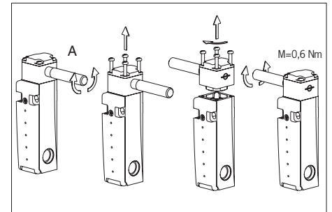
Fig. 1 : Changement de la direction d'actionnement
