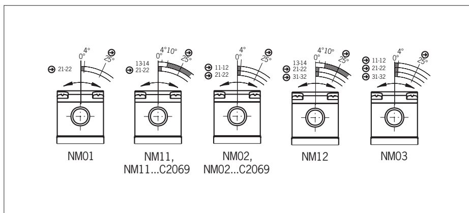
Fig. 4 : Diagrammes de commutation NM..AV/NM..AL
