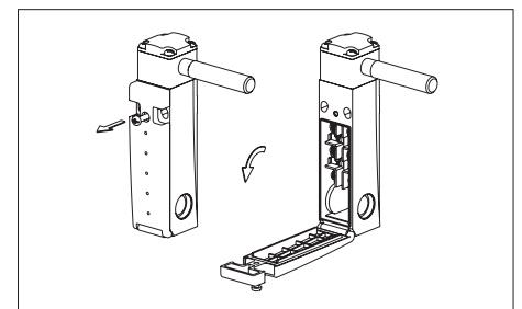
Fig. 2 : Ouverture de l'interrupteur de sécurité
