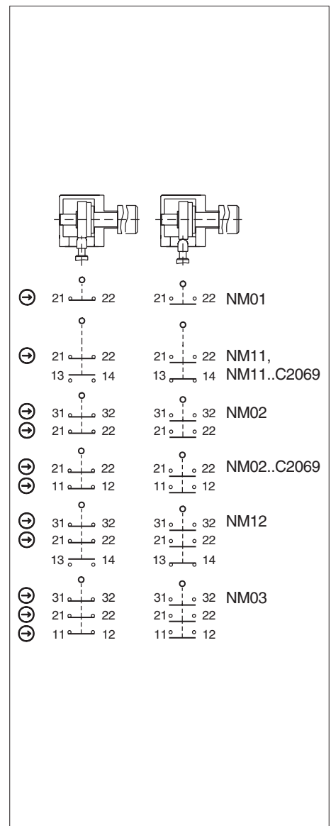
Fig. 3 : Éléments de commutation et fonctions de commutation
