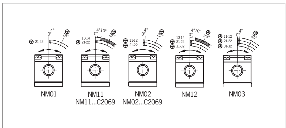
Fig. 4 : Diagrammes de commutation NM..AK/NM..AG
