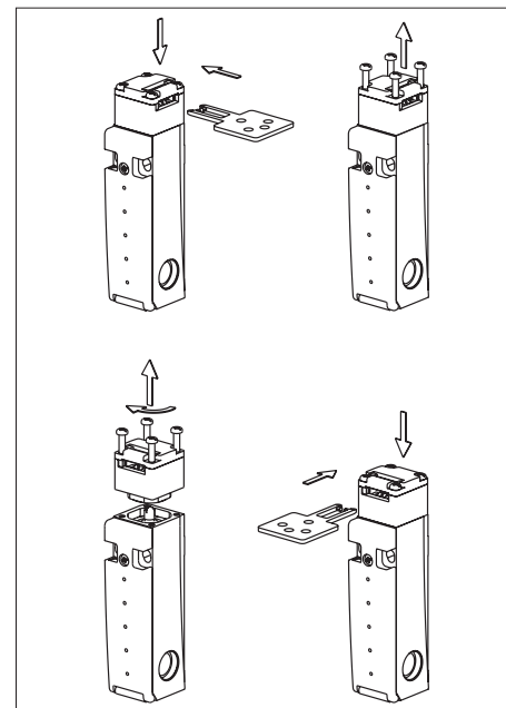
Fig. 1 : Changement de la direction d'actionnement
