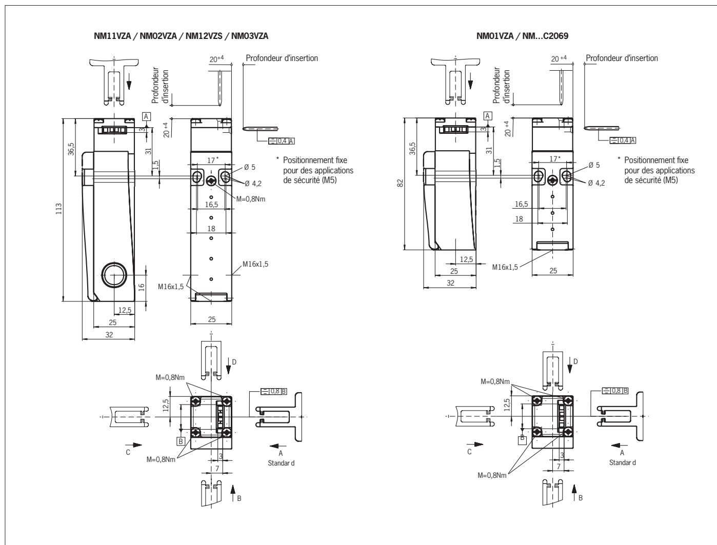
Fig. 4 : Dimensions NM...
