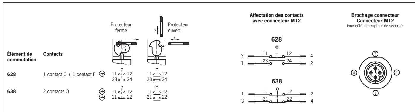
Fig. 4 : Éléments de commutation et fonctions de commutation
