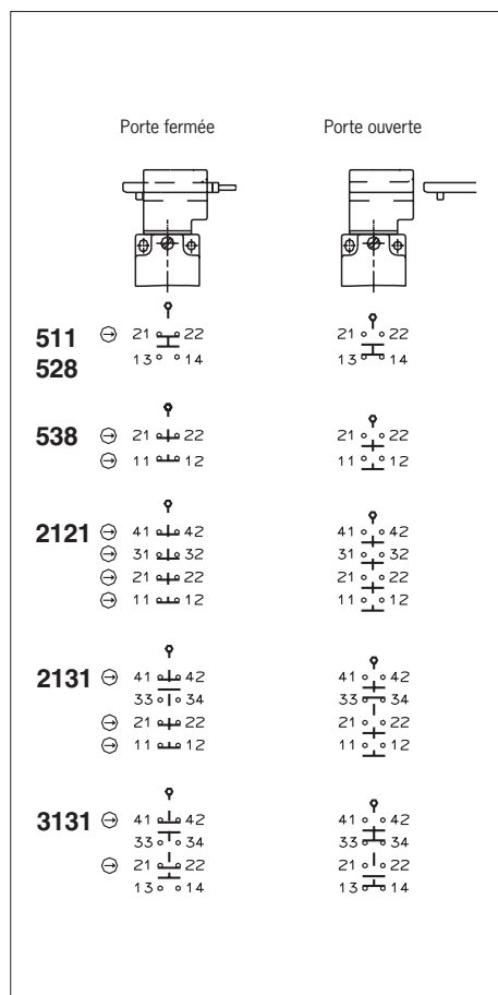
Fig. 2 : Éléments de commutation et fonctions de commutation
