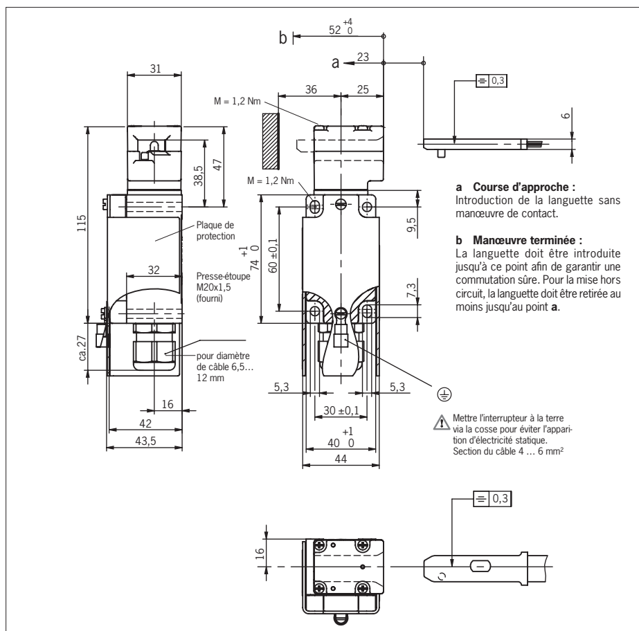
Fig. 3 : Dimensions NZ1VZ...EX
