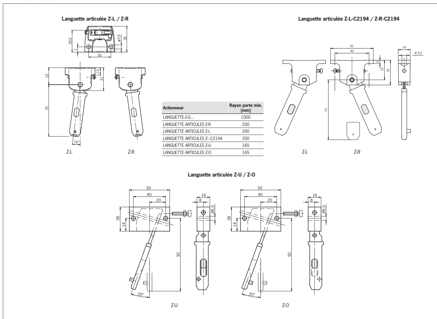
Fig. 4 : Rayons de porte minimum
