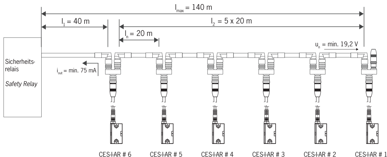
Figure 1 : Exemple de câblage avec six CES-I-AR
