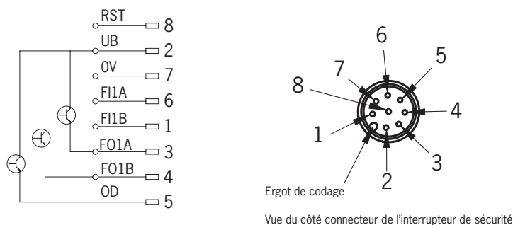
Figure 2 : Affectation des broches interrupteur de sécurité CES-I-AR
