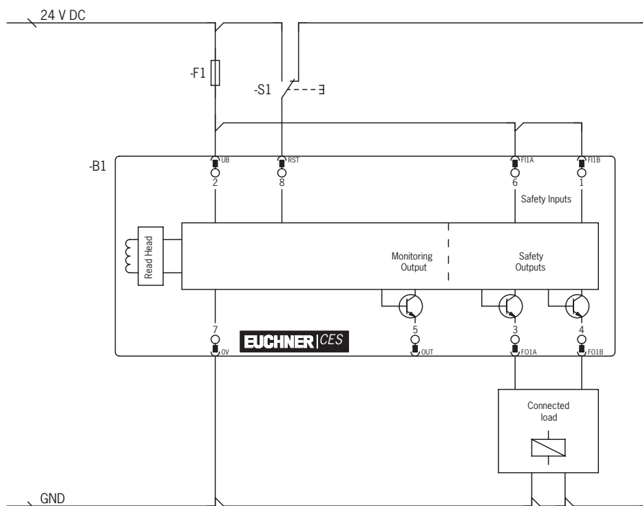
Figure 3 : Exemple de raccordement interrupteur individuel CES-I-AR...
