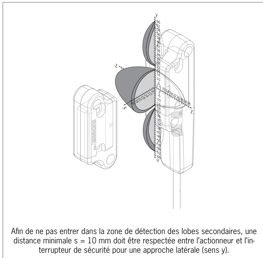
Figure 5 : Zone de détection type
