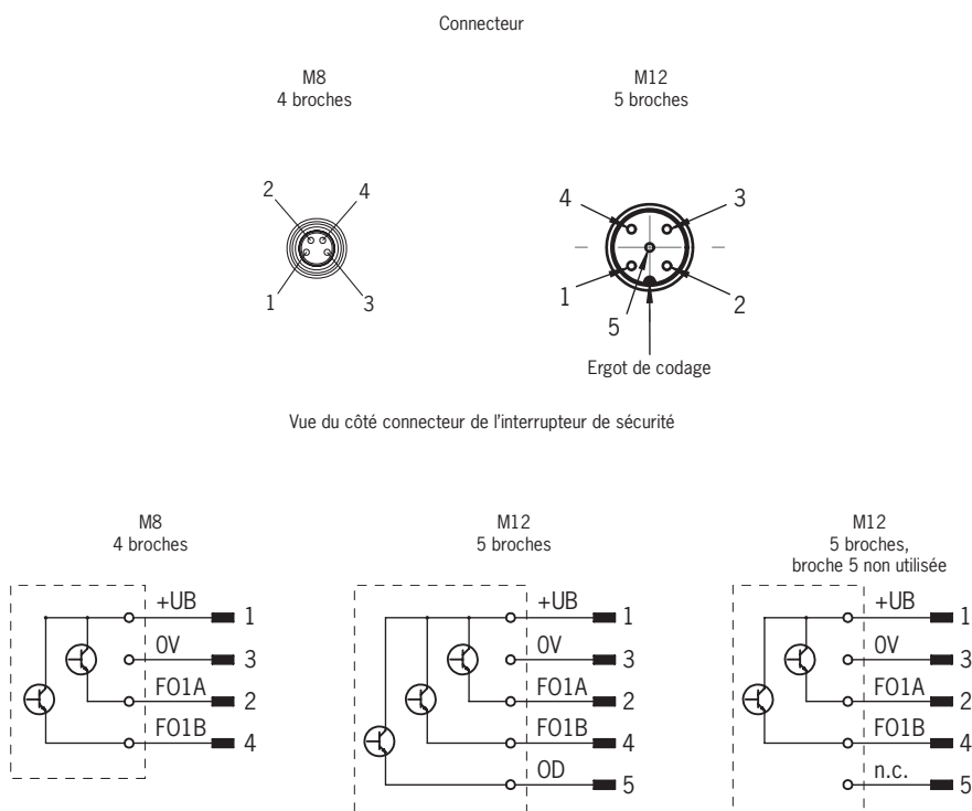
Figure 1 : Affectation des broches interrupteur de sécurité CES-I-AP-.-C04
