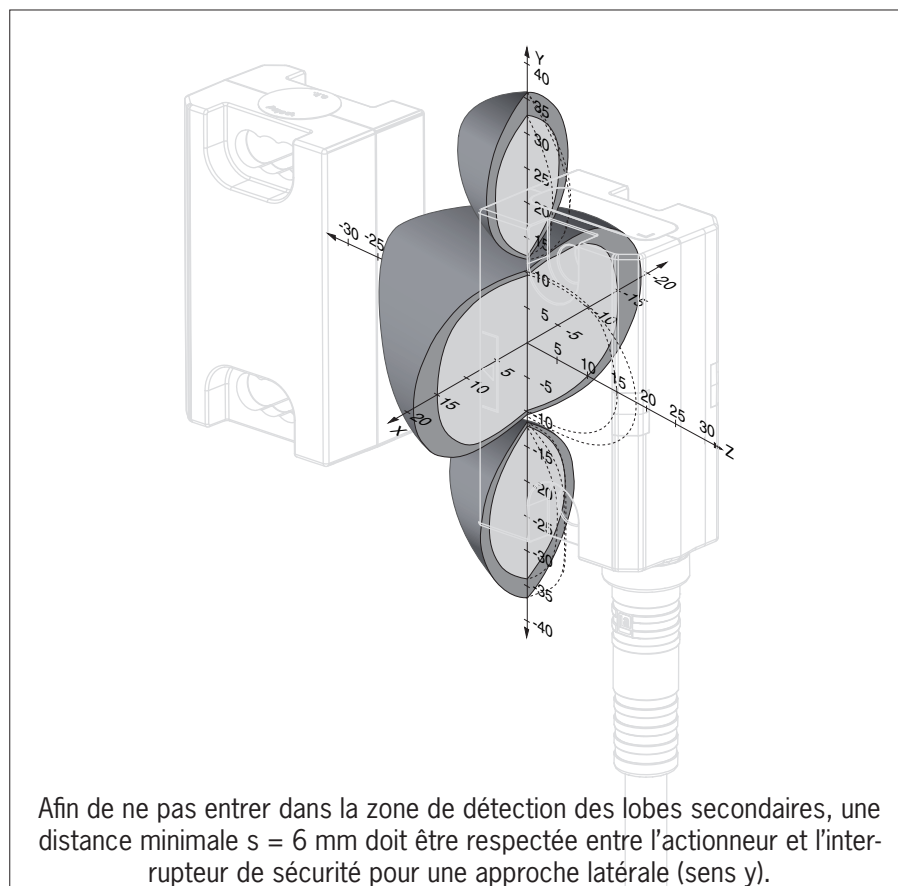
Figure 4 : Zone de détection type
