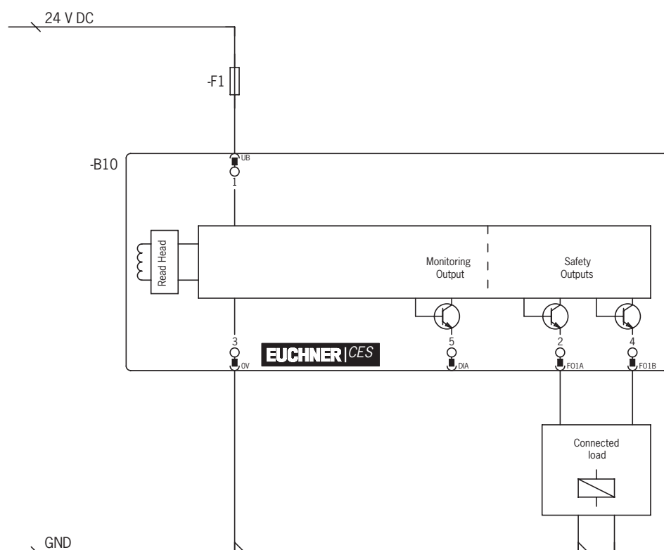
Figure 2 : Exemple de raccordement CES-I-AP-...
