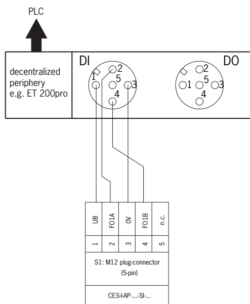
Figure 3 : Exemple de raccordement version pour modules d'interfaces décentralisées
